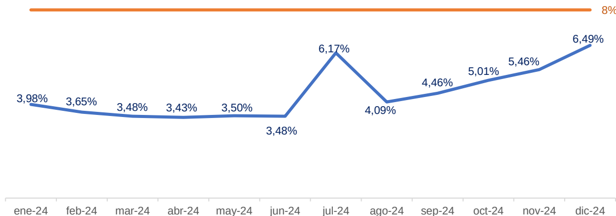
Gráfico No. 5: Valor en Riesgo (VaR)
