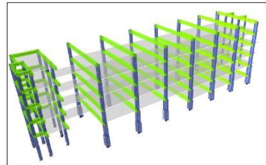
Modelo Tridimensional Torre Occidental
