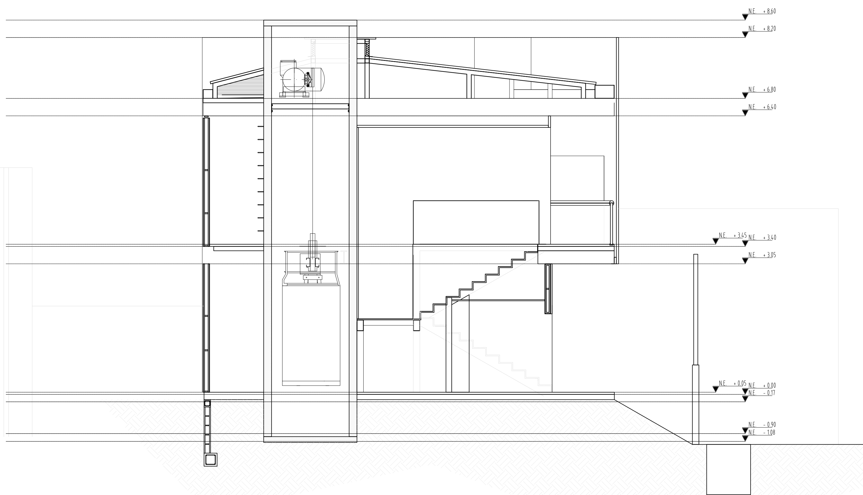
CORTE C-C' | TRANSVERSAL SOBRE ESCALERA
