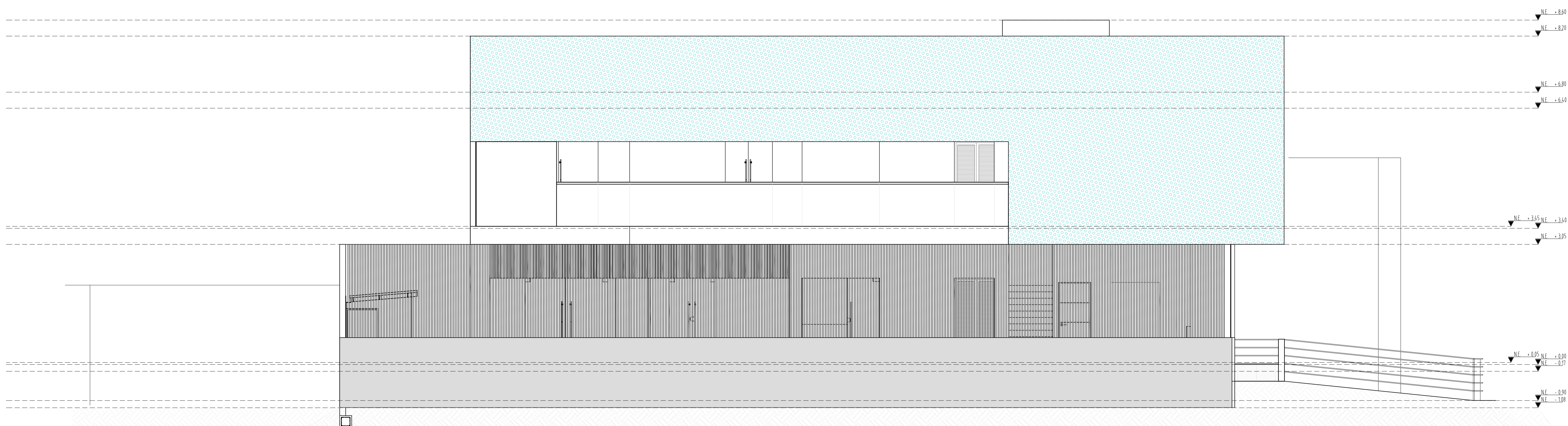
FACHADA ESTE CON CERRAMIENTO
