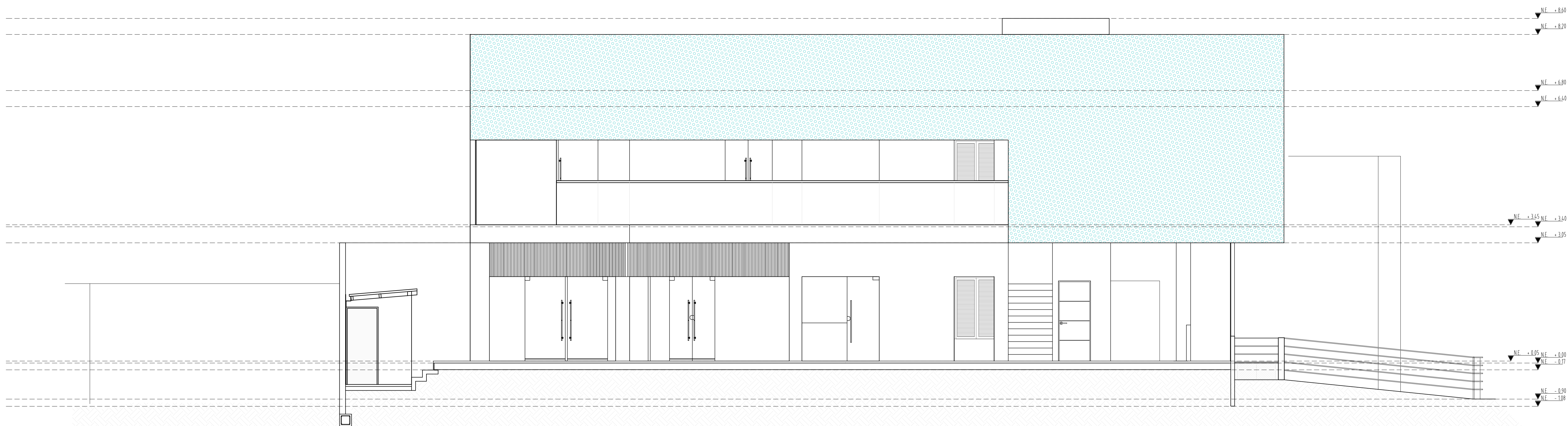
FACHADA ESTE SIN CERRAMIENTO
