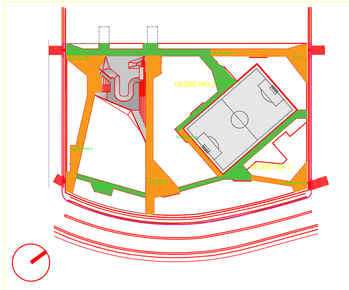
LUPA PLANTA MANZANA 14 - ESCALA 1:100 (VER: DET-013P en escala 1:250)
