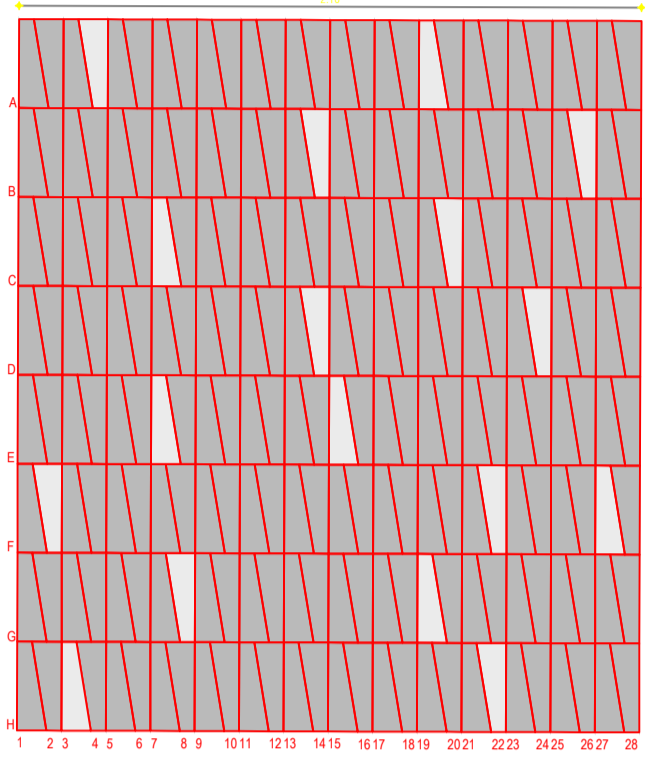
MODULO PISOS EN ADOQUIN ESCALA 1:20
