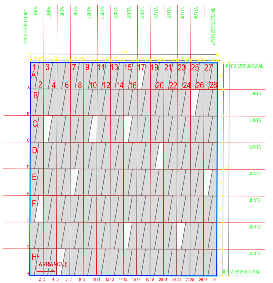
MODULO PISOS EN ADOQUIN ESCALA 1:20
