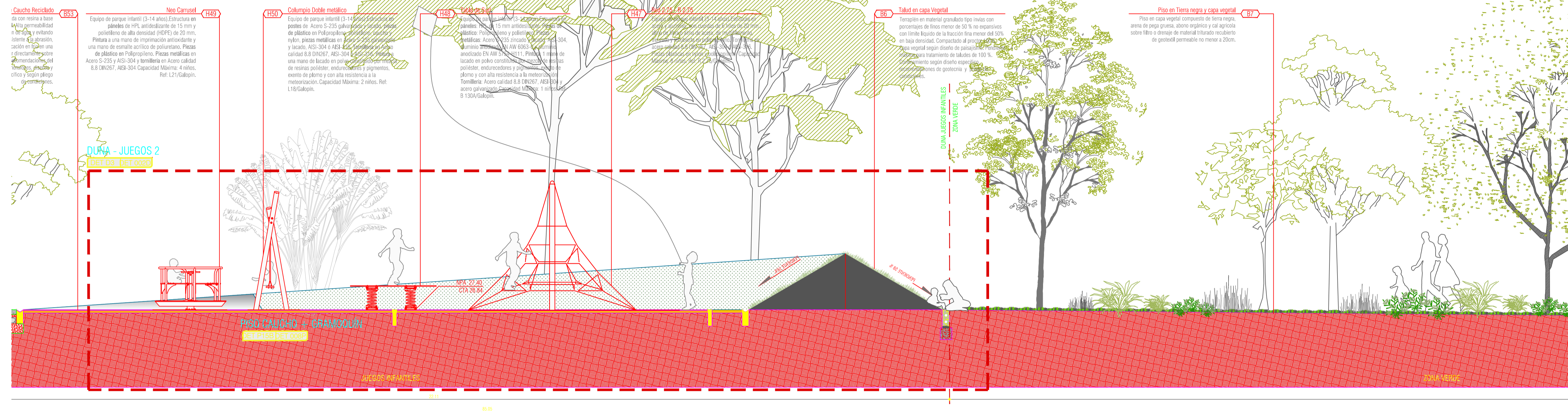
SECCIÓN 5 (SUROCCIDENTE - NORORIENTE) MANZANA 20 PARQUE RECREO DEPORTIVO VILLAS DE SAN PABLO ESCALA 1:50
