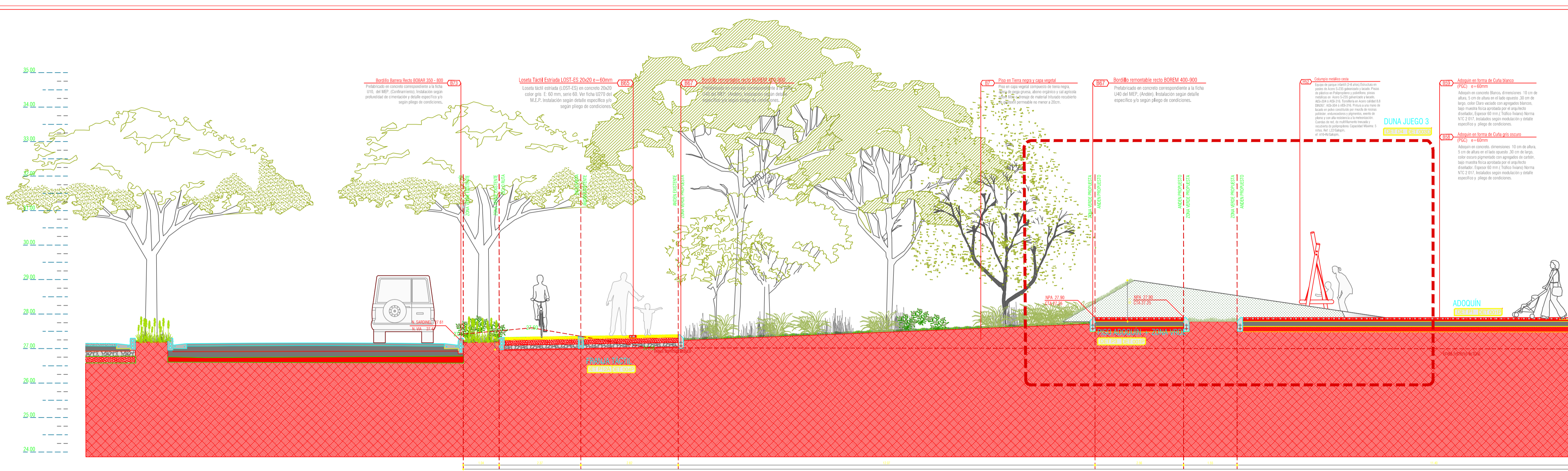
SECCIÓN 1 (NORTE-SUR) - MANZANA 14 PARQUE RECREO DEPORTIVO VILLAS DE SAN PABLO ESCALA 1:50
