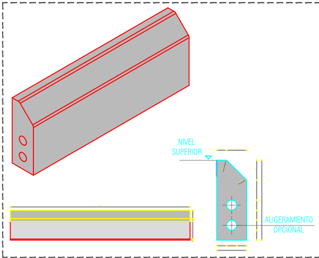
B67 Bordillo remontable recto BOREM 400-900
