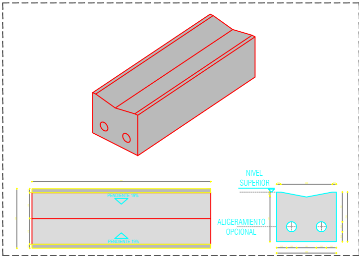
B69 Cuneta Auxiliar Serie 250 Confinamiento de Pavimentos Segmentados
