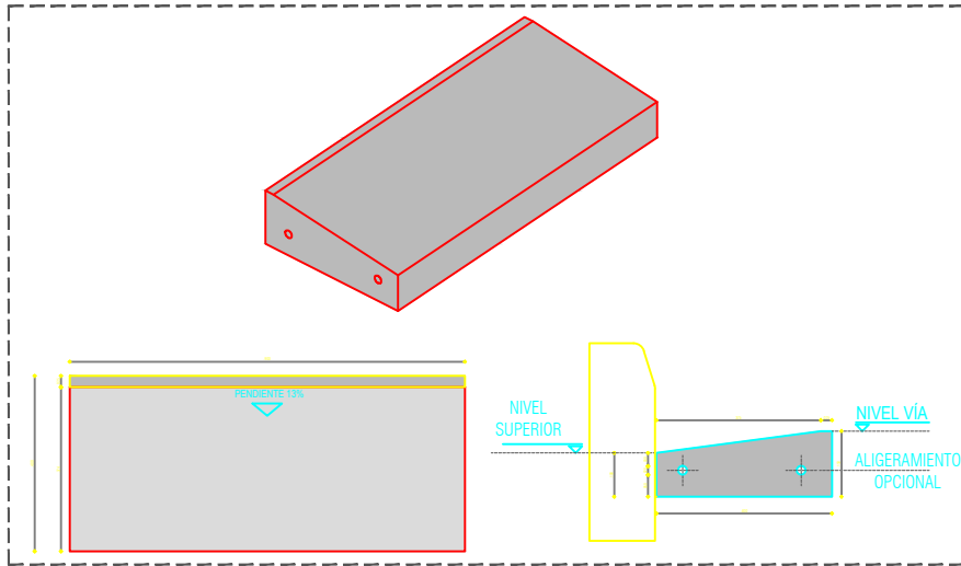
B68 Cuneta Vial CUVIA 150-900
