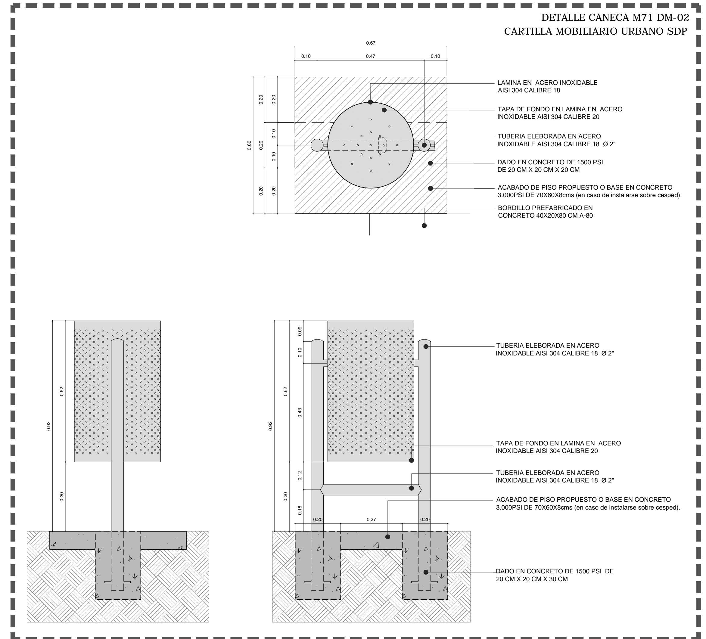
CANECA ACERO INOXIDABLE M71 Esc. 1:10
