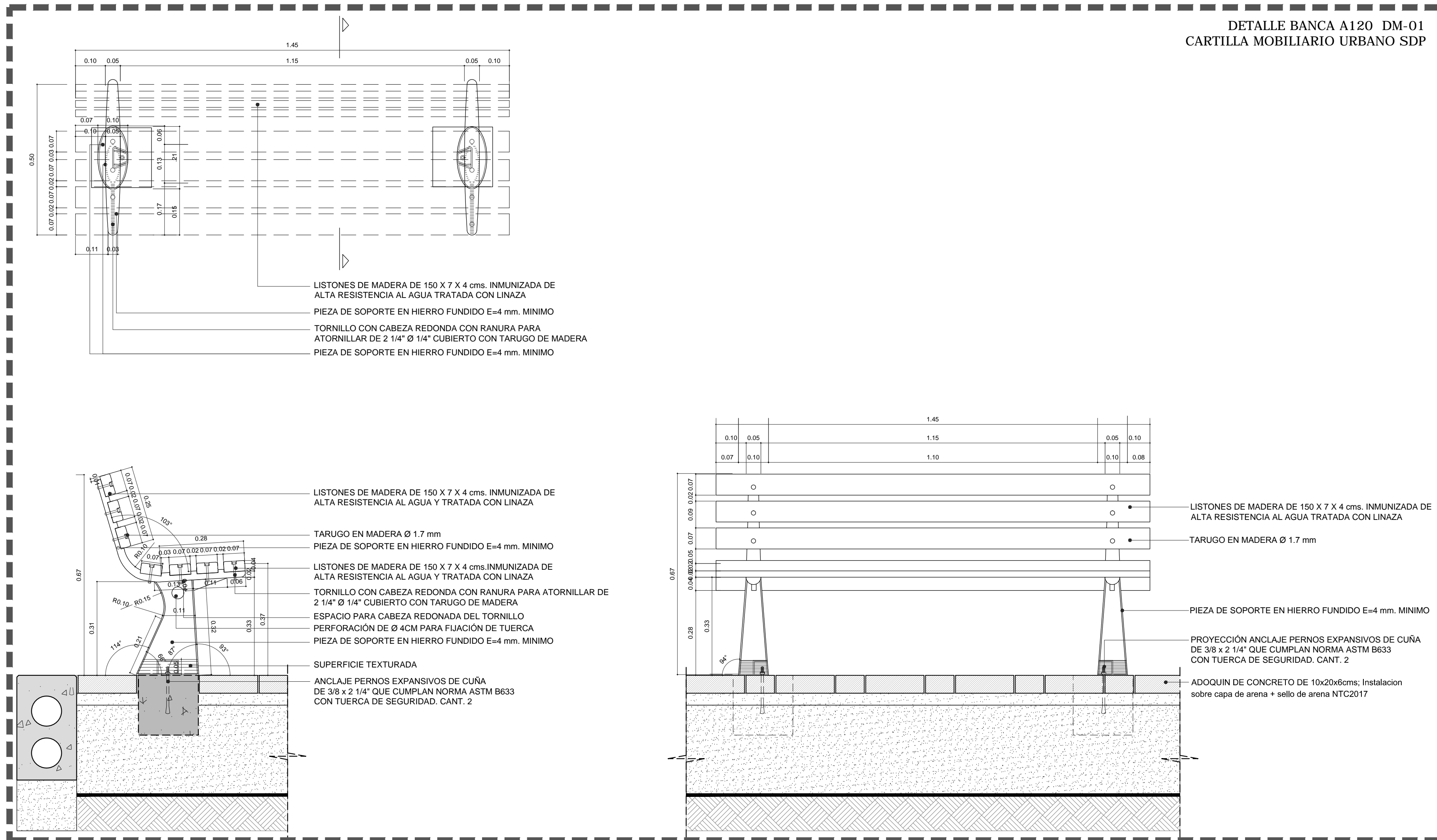
BANCA MADERA A-120 Esc. 1:10
