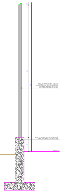
DETALLE 6 - PÁRALES VERTICALES - TIPO B ALZADO INTERIOR CANCHA MULTIPLES ESC. 1_20
