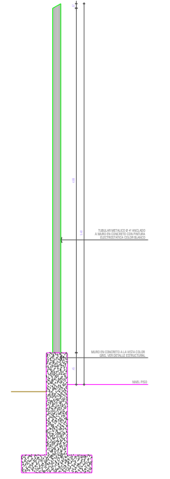
DETALLE 6 - PÁRALES VERTICALES - TIPO C ALZADO INTERIOR CANCHA MULTIPLES ESC. 1_20
