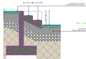
DETALLE 3 - FIELDADO EN CONCRETO COSTE ESC. 1_20
