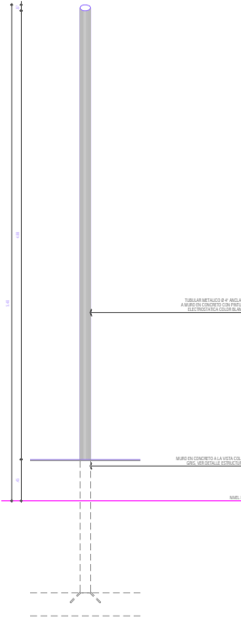
DETALLE 6 - PÁRALES VERTICALES - TIPO C ALZADO INTERIOR CANCHA MULTIPLES ESC. 1_20
