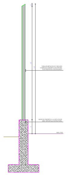
DETALLE 6 - PÁRALES VERTICALES - TIPO A ALZADO INTERIOR CANCHA MULTIPLES ESC. 1_20
