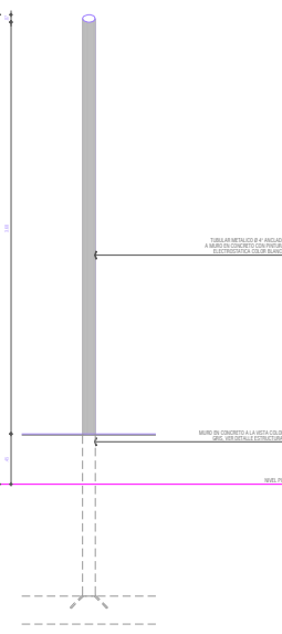
DETALLE 6 - PÁRALES VERTICALES - TIPO B ALZADO INTERIOR CANCHA MULTIPLES ESC. 1_20
