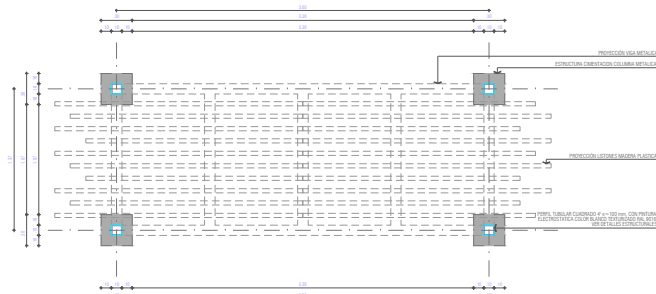
DETALLE 2 - PERILLA TIPO PLANTA COLUMNAS ESC. 1 / 20
