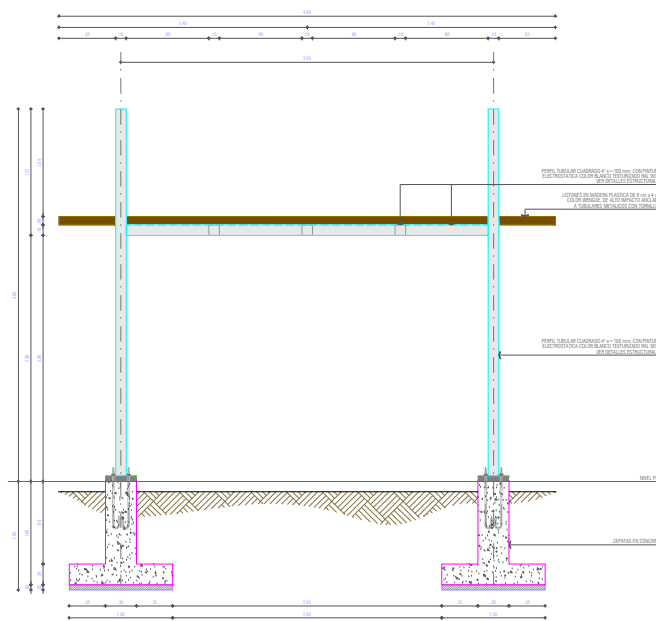
DETALLE 7 - PERILLA TIPO ALZADO GENERAL ESC. 1 / 20
