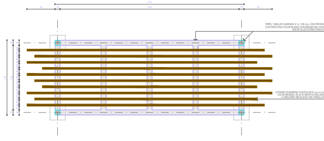
DETALLE 2 - PERILLA TIPO CORTADO ESC. 1 / 20
