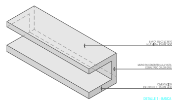
DETALLE 1 - BANCA ALZADO GENERAL ESC. 1 / 20
