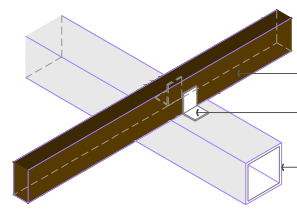
DETALLE 2 - PERILLA TIPO CORTADO ESC. 1 / 5
