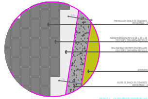
DETALLE - 18 DESPESE ADOQUIN #3 PLANTA ESC 1/10
