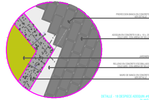
DETALLE - 18 DESPESE ADOQUIN #6 PLANTA ESC 1/10
