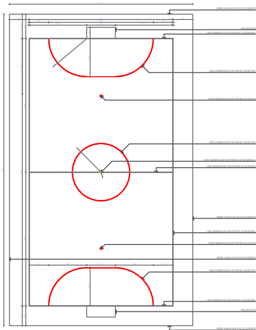
DETALLE - 19 SEÑALIZACION CANCHA MICROFUTBOL ESC 1/100
