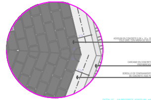
DETALLE - 18 DESPESE ADOQUIN #7 PLANTA ESC 1/10
