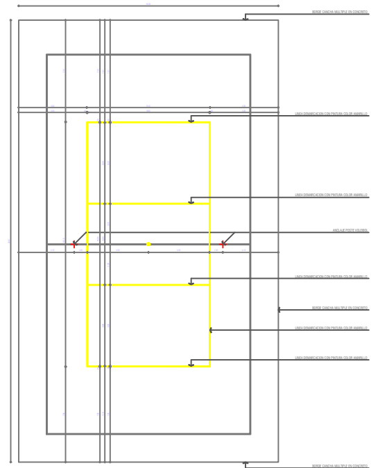
DETALLE - 19 SEÑALIZACION CANCHA VOLEIBOL ESC 1/100
