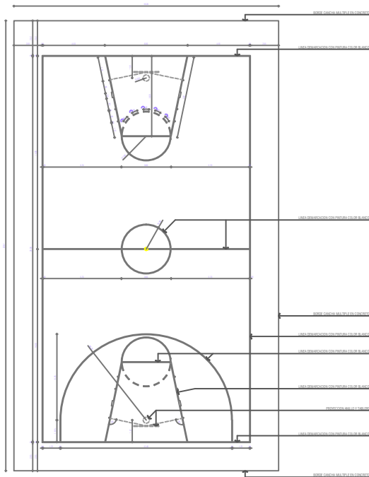
DETALLE - 19 SEÑALIZACION CANCHA BASKETEBOL ESC 1/100
