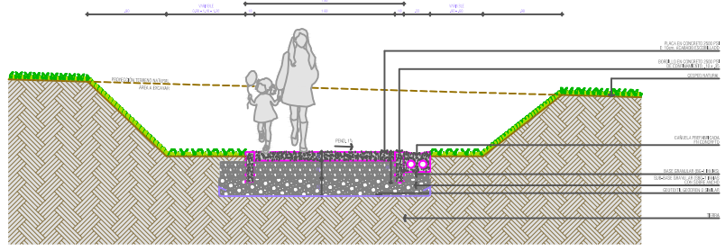
DETALLE 12 - SENDERO PEATONAL CON CAJILLA ESC. 1/10
