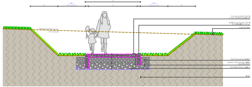
DETALLE 12 - SENDERO PEATONAL CON CAJILLA ESC. 1/10
