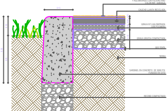
DETALLE 11 - BORDILLO PISO CAUCHO - AREA PAVIMENTADA ESC. 1/10
