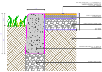
DETALLE 11 - BORDILLO PISO CAUCHO - BORDILLO ALEROS ESC. 1/10
