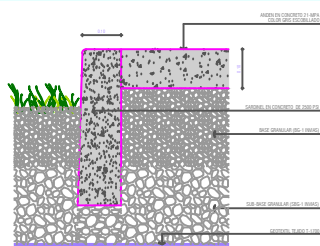
DETALLE 11 - BORDILLO AREA EN CONCRETO ESC. 1/10
