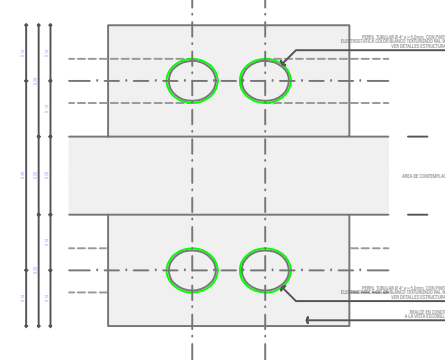
DETALLE 2 - PERIFERIA - REAL DE TUBERIAS DE AGUAS ESC: 1/5
