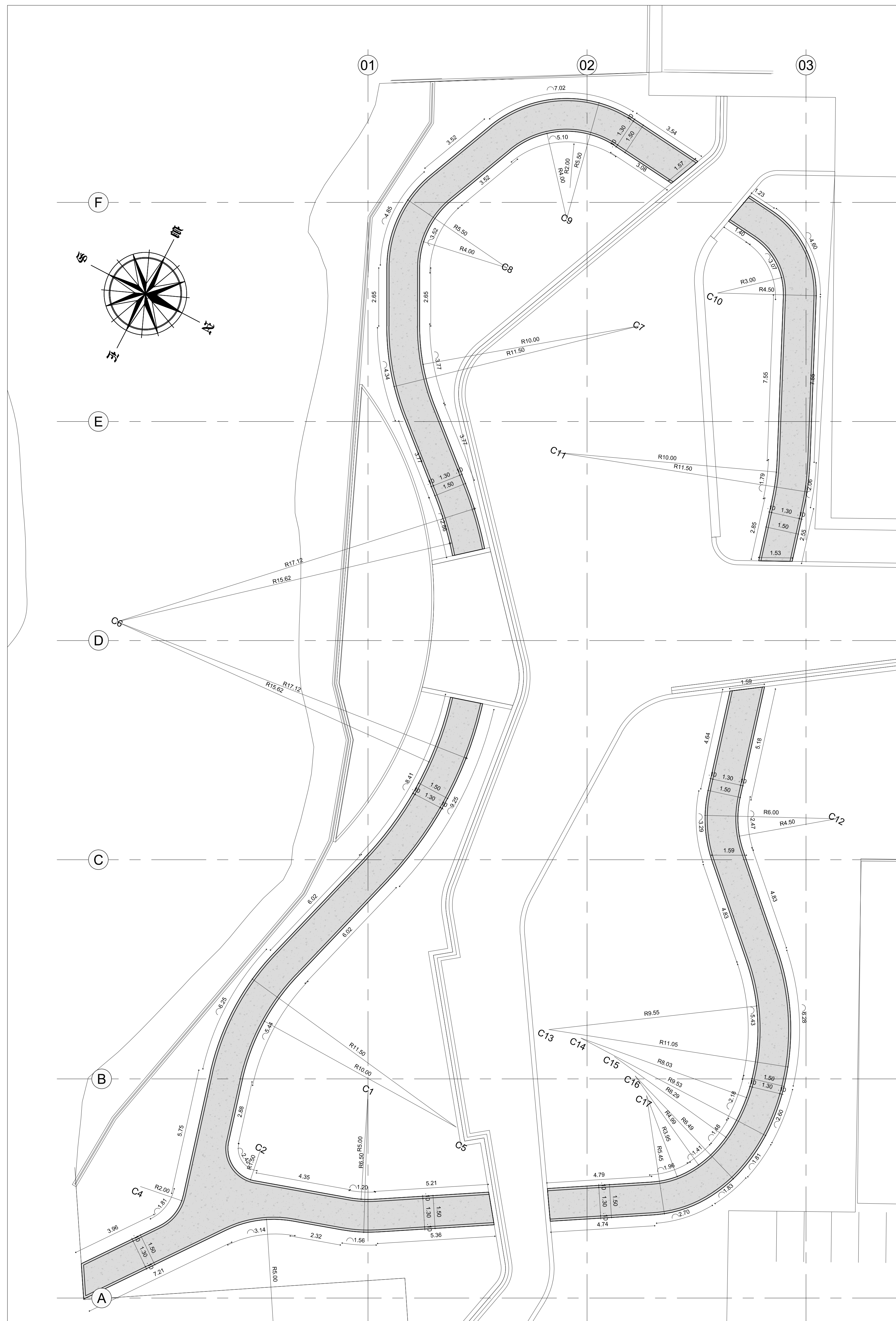
PISTA DE TROTE-PLANTA DE GEOMETRIA Esc. 1:100
