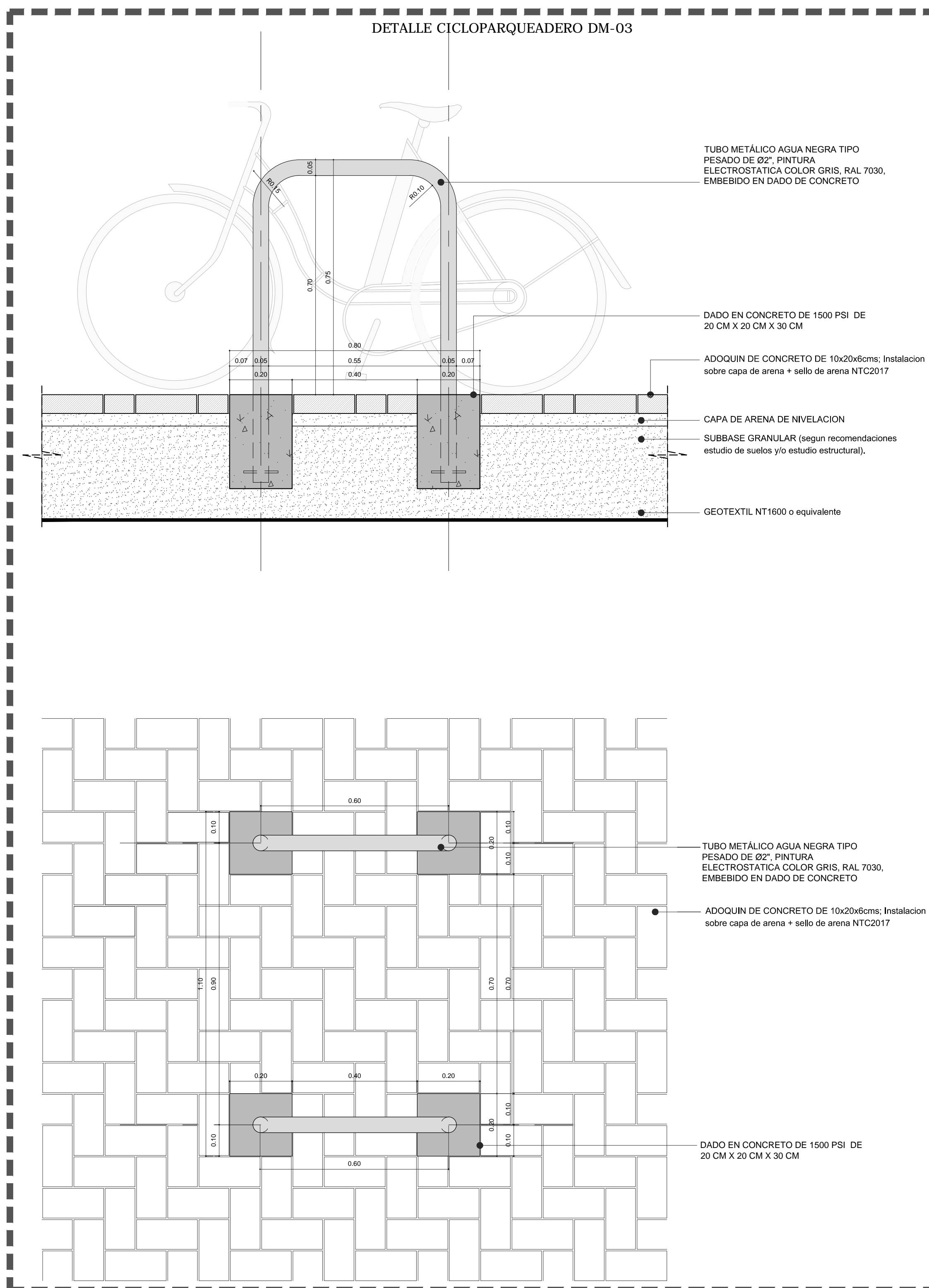
CICLOPARQUEADERO Esc. 1:10
