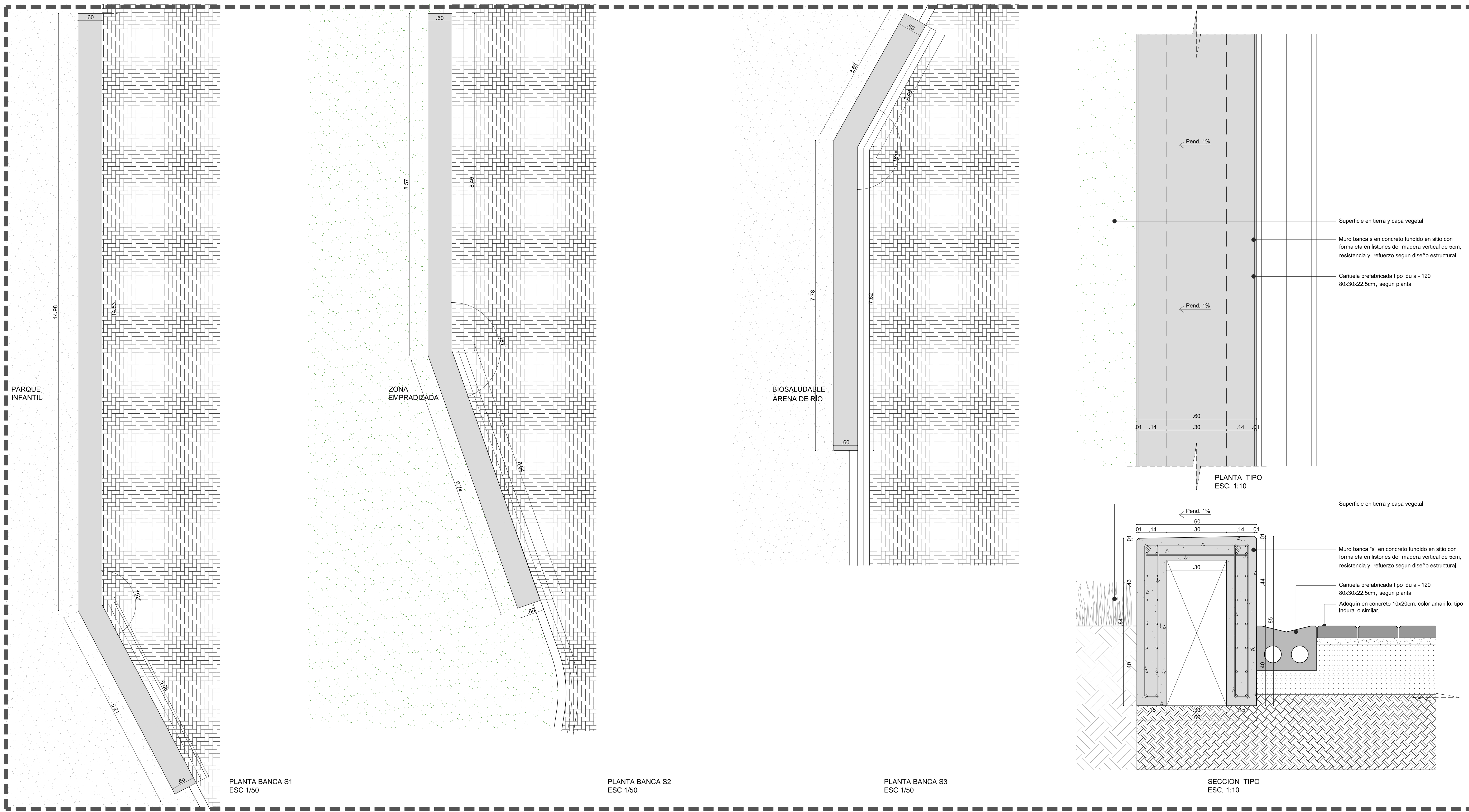
DETALLE BANCA S1, S2 Y S3
