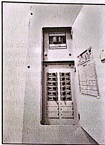
Ilustración 5 Tablero de circuitos instalado con breakers
