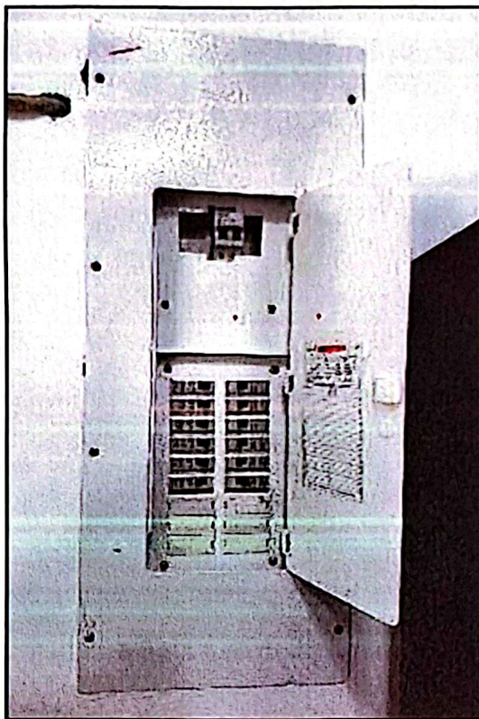
Ilustración 6 Tablero de distribución eléctrica
