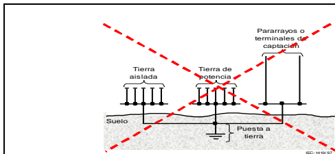
Figura 15.3. Una sola puesta a tierra para todas las necesidades
