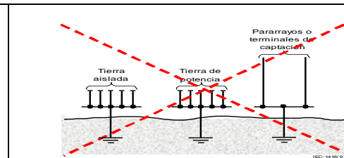
Figura 15.2. Puestas a tierra separadas o independientes
