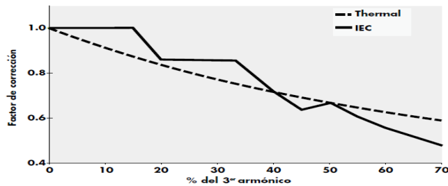
Figura 13 - Factor de corrección en función de la proporción del contenido de armónicos triple-N
