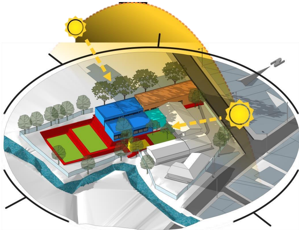
Cubiertas inclinadas para evitar radiación y manejo de lluvia.
