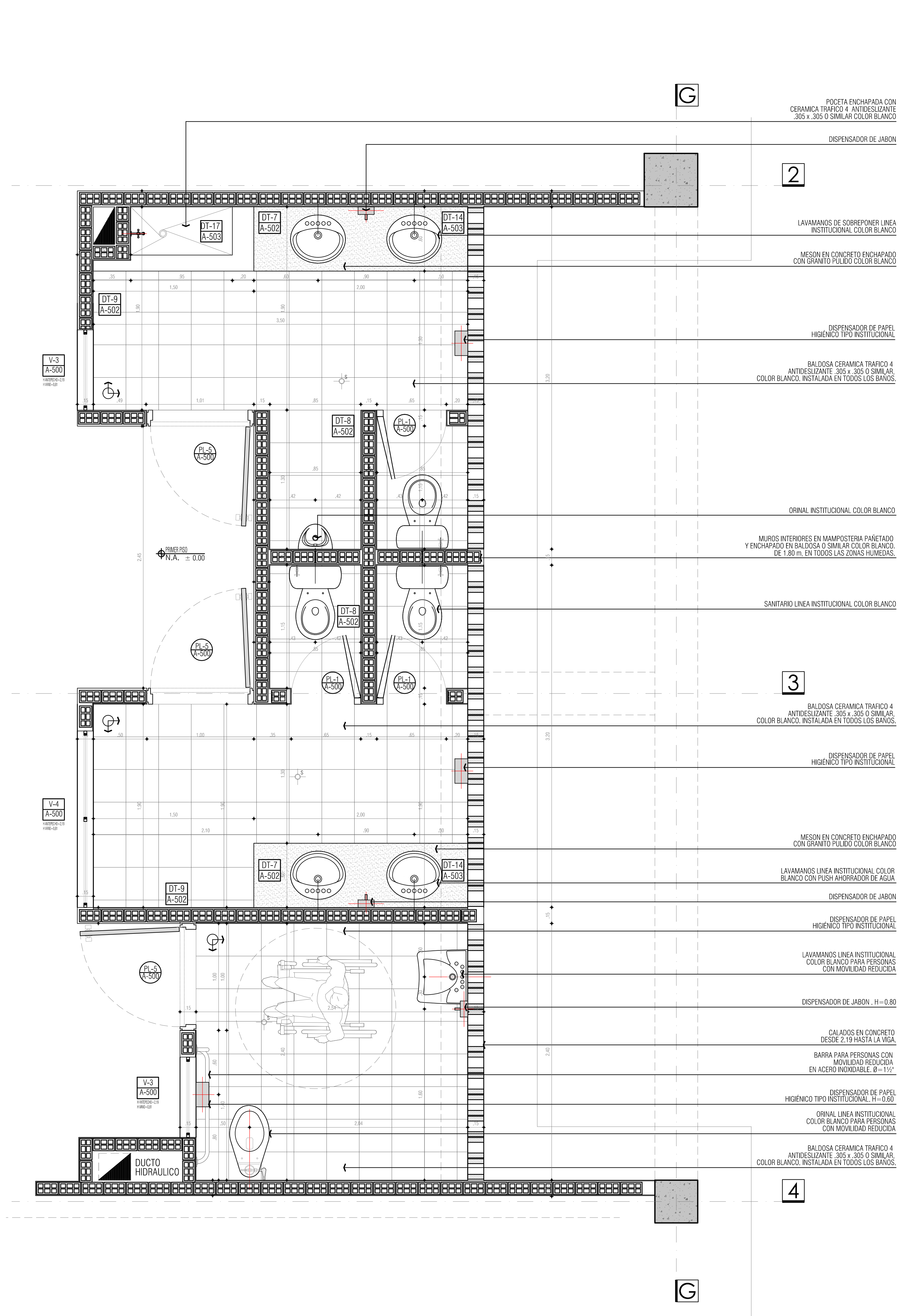
I.E. AGROECOL SAN RAFAEL CHOCÓ DETALLE BAÑOS ESC 1_20
