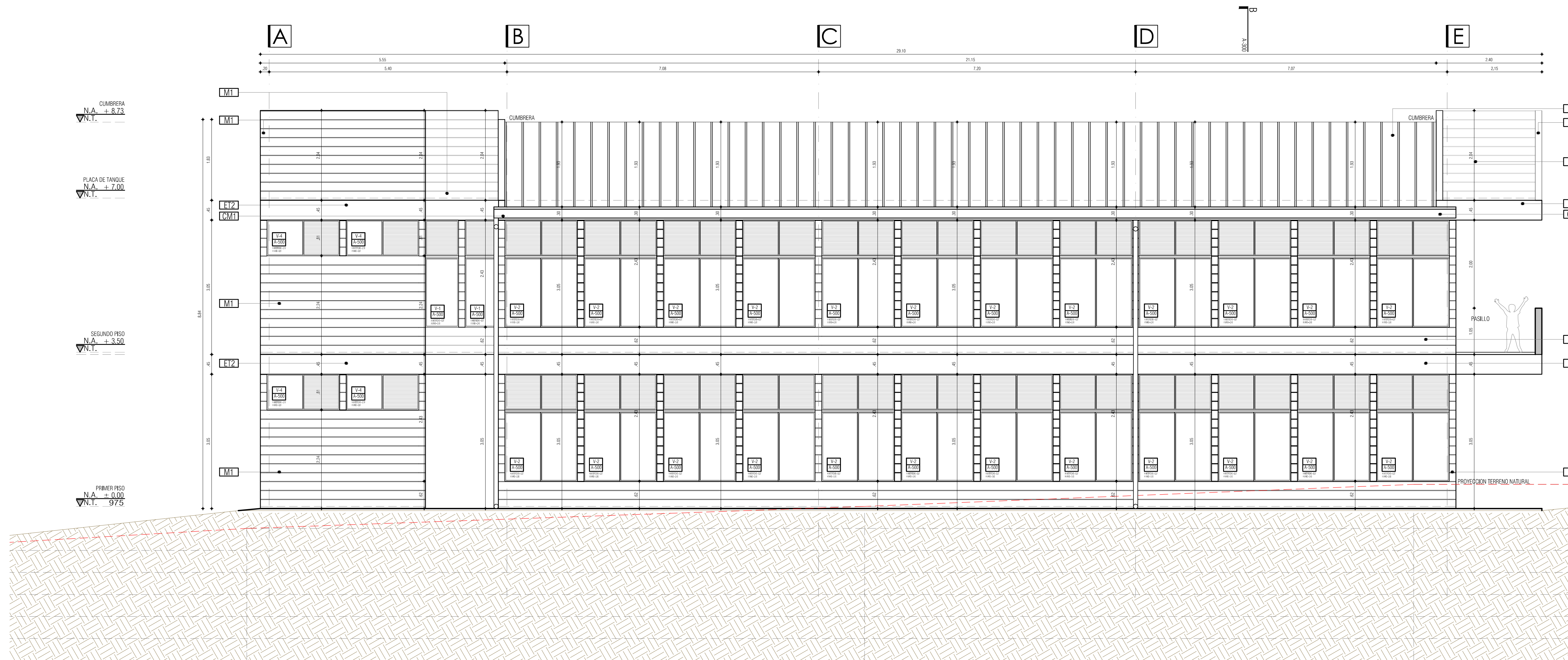
I.E. SANTA TERESITA DE ALTAQUER PASTO FACHADA SUR MÓDULO A ESC 1_50
