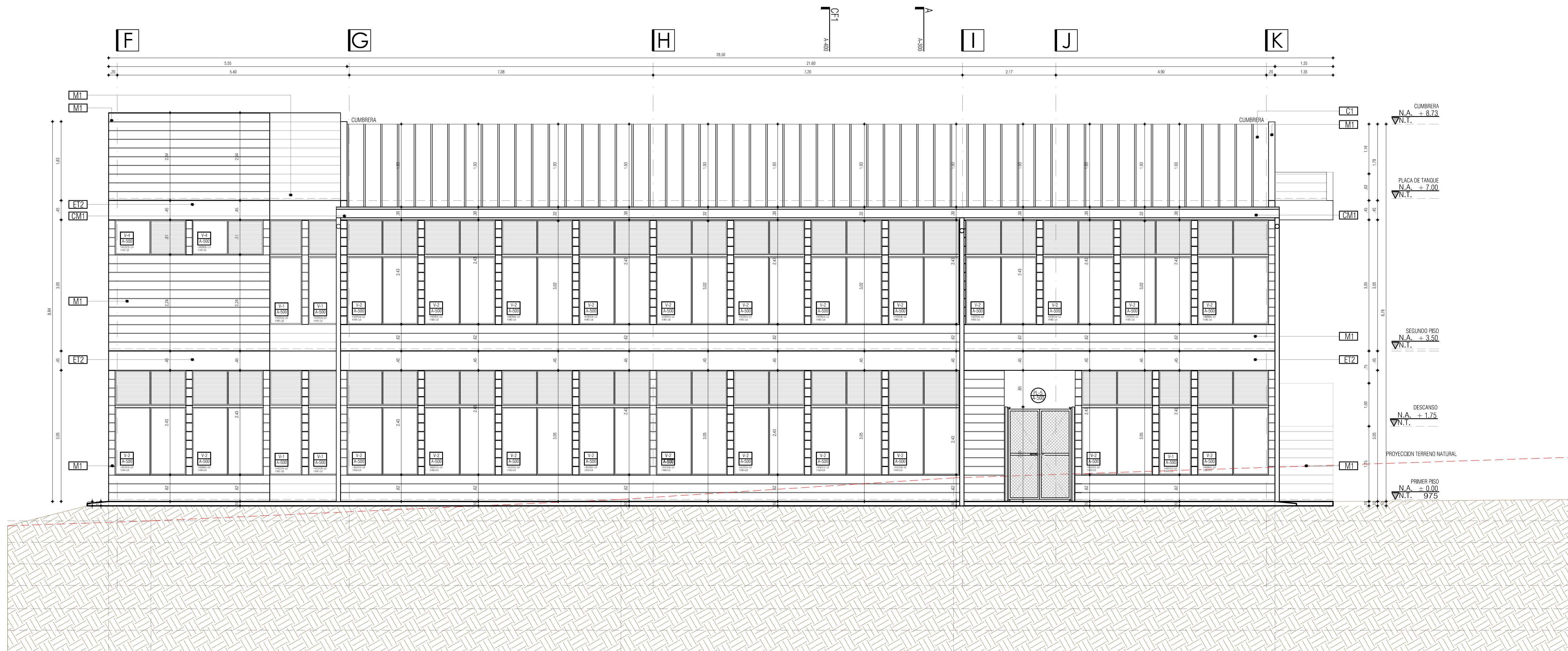
I.E. SANTA TERESITA DE ALTAQUER PASTO FACHADA SUR MÓDULO B ESC 1_50
