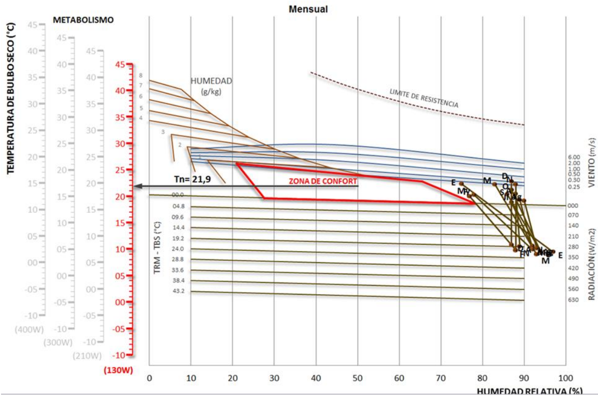
Grafica 6 Carta Bioclimática
