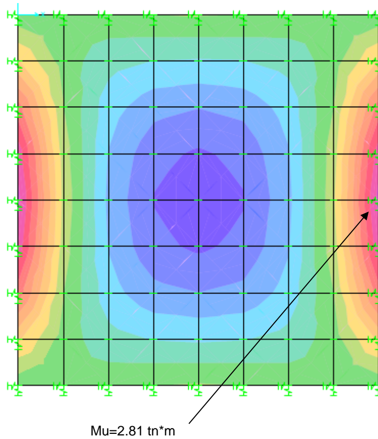
FIGURA 12. DIAGRAMA DE MOMENTO M1-1 – LOSA DE FONDO
