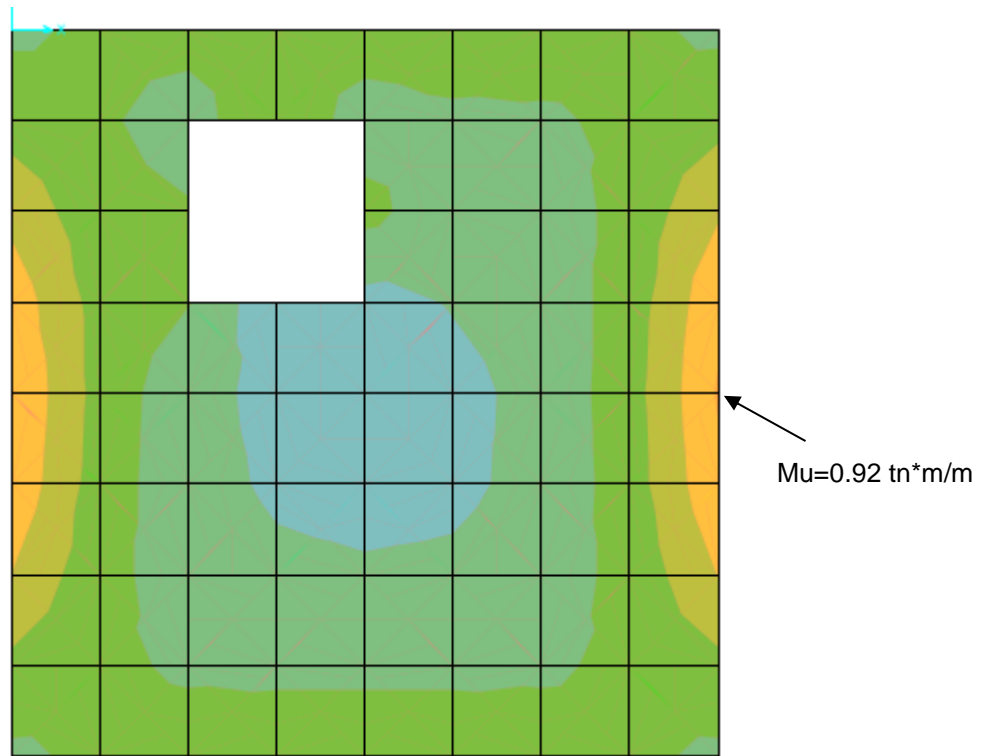
FIGURA 14. DIAGRAMA DE MOMENTO M1-1 – Losa Superior
