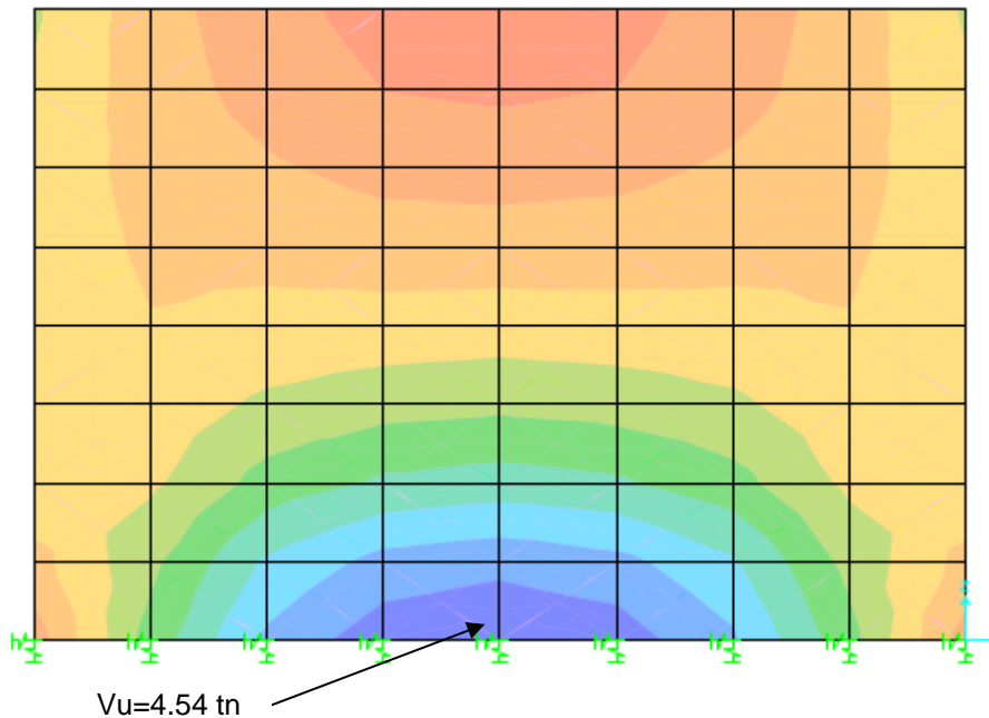
FIGURA 9. DIAGRAMA DE CORTANTE V23 – MURO 1
