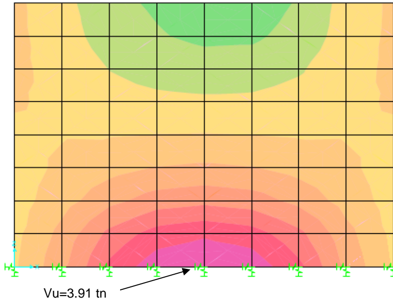
FIGURA 11. DIAGRAMA DE CORTANTE V23 (COMBO 3) MURO 2
