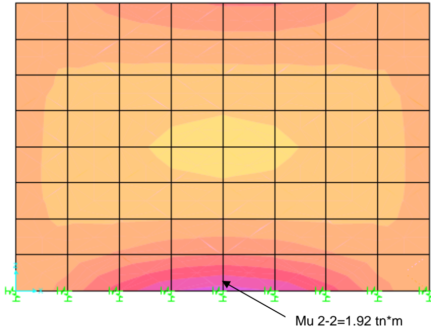
FIGURA 10. DIAGRAMA DE MOMENTO M2-2 (COMBO 3) MURO 2
