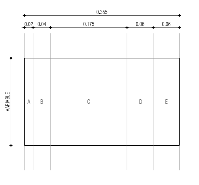
DETALLE 4 - ALFAJA Y FLANQUE METÁLICO DESARROLLO - PLANTA ESC 1_5
