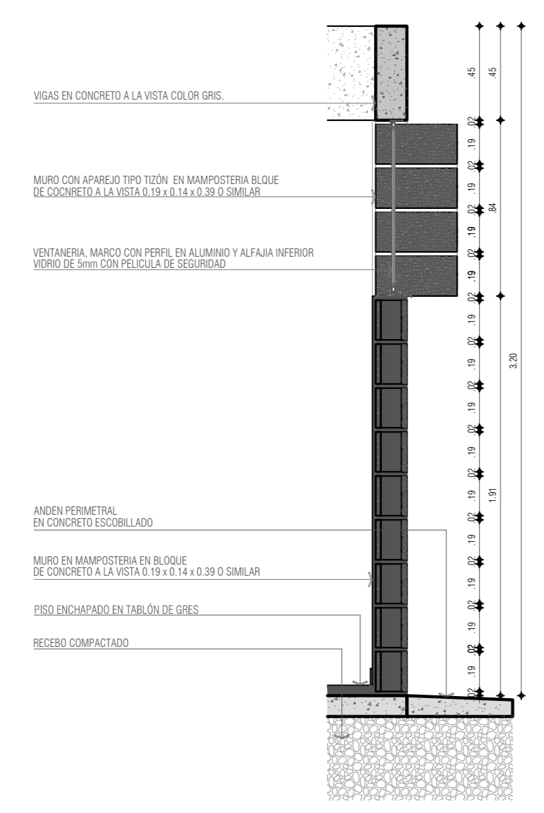
DETALLE 2 - MACHÓN VENTANA TIPO 2 CORTE ESC 1_20
