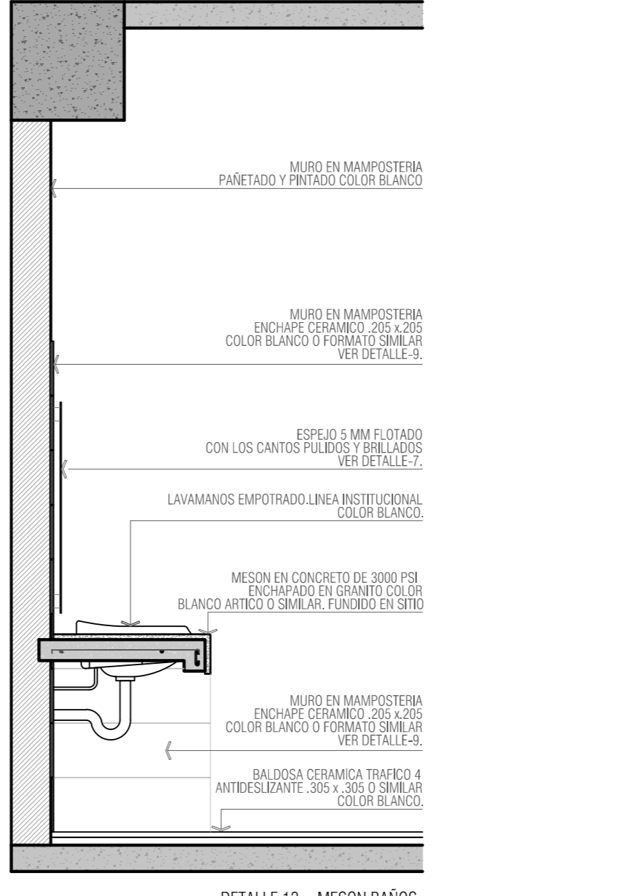
DETALLE 12 - MESÓN BAÑOS LABORATORIO CORTE ESC 1_20
