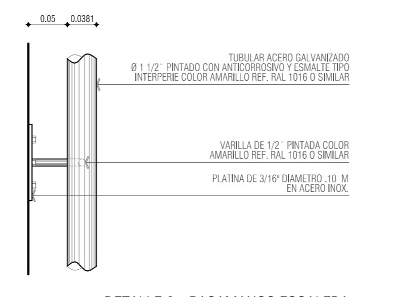
DETALLE 8 - PASAMANOS ESCALERA PLANTA ESC 1_5
