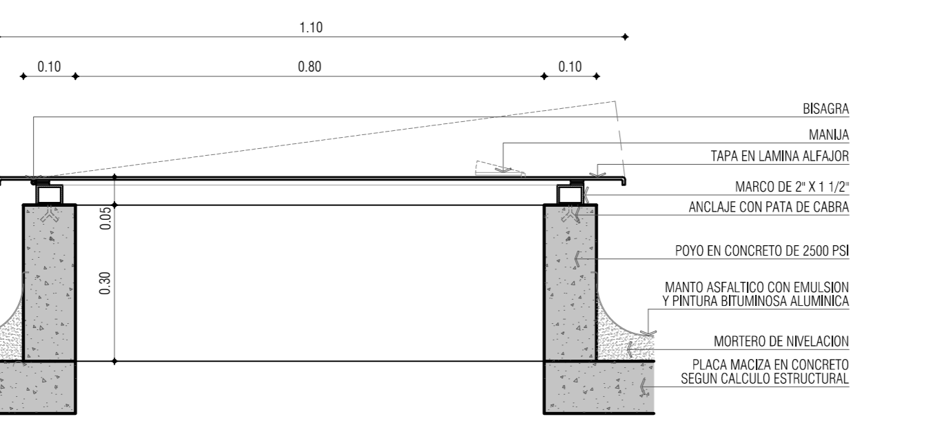
DETALLE 11 - ESCOTILLA CORTE ESC 1_10
