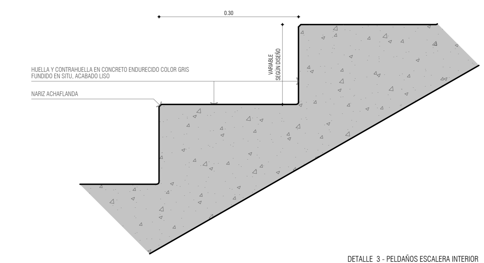
DETALLE 3 - PELDAÑOS ESCALERA INTERIOR CORTE ESC 1_5
