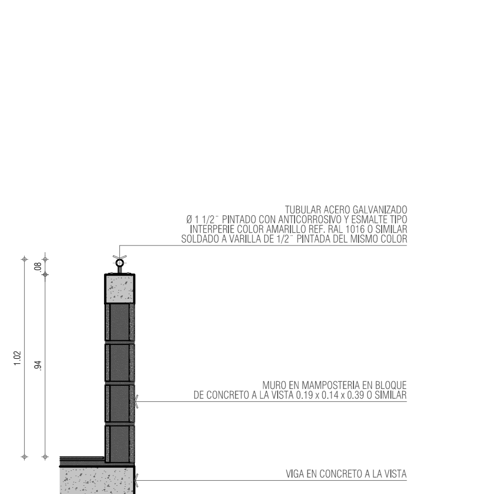
DETALLE 10 - ANTEPECHO CIRCULACIONES CORTE ESC 1_20
