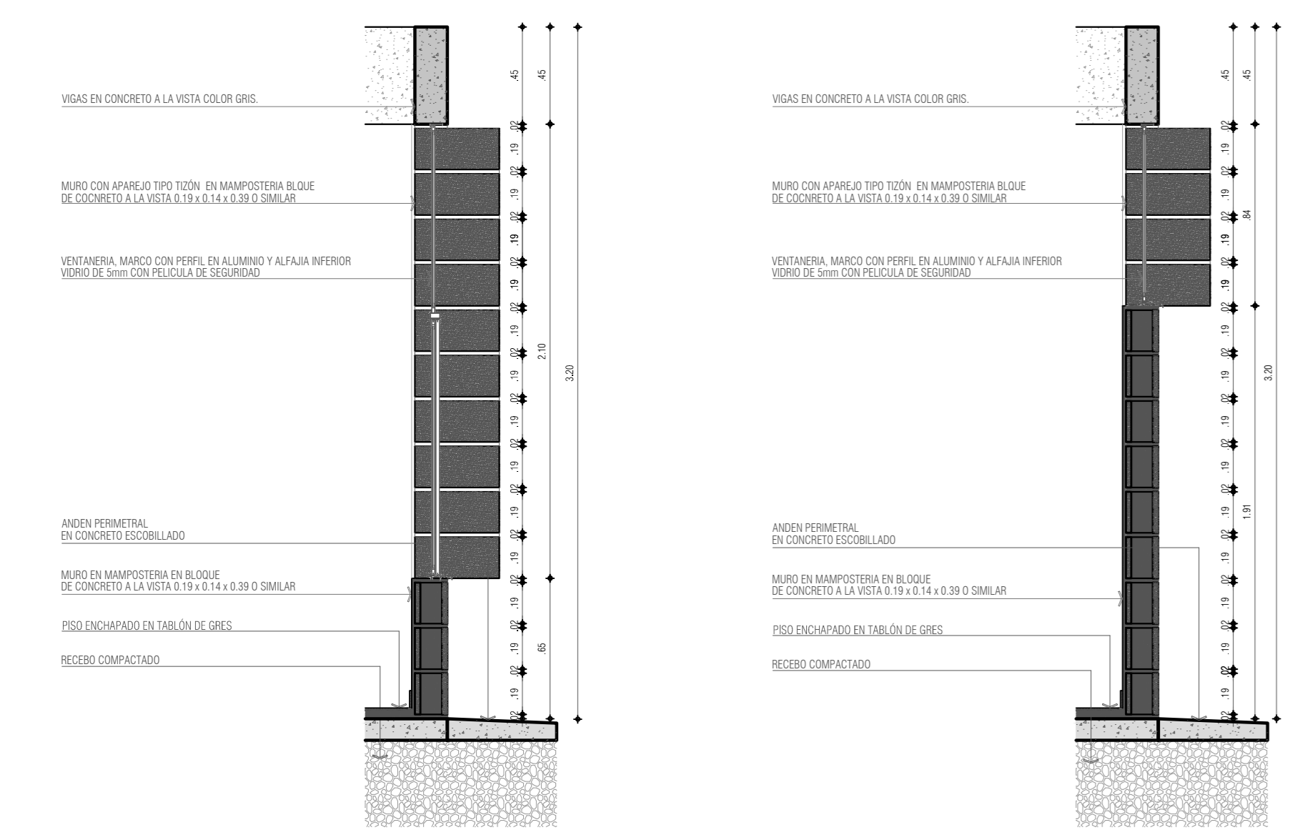
DETALLE 1 - MACHÓN VENTANA TIPO 1 CORTE ESC 1_20
