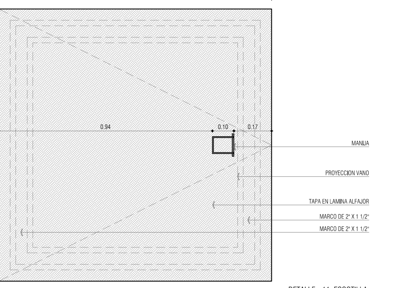
DETALLE 11 - ESCOTILLA PLANTA ESC 1_10
