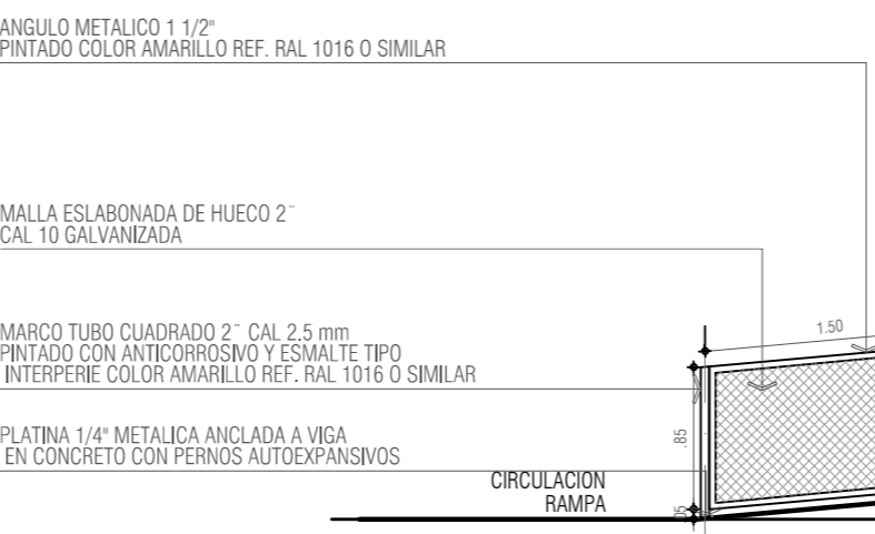
DETALLE 9 - BARANDA RAMPA ALZADO ESC 1_50
