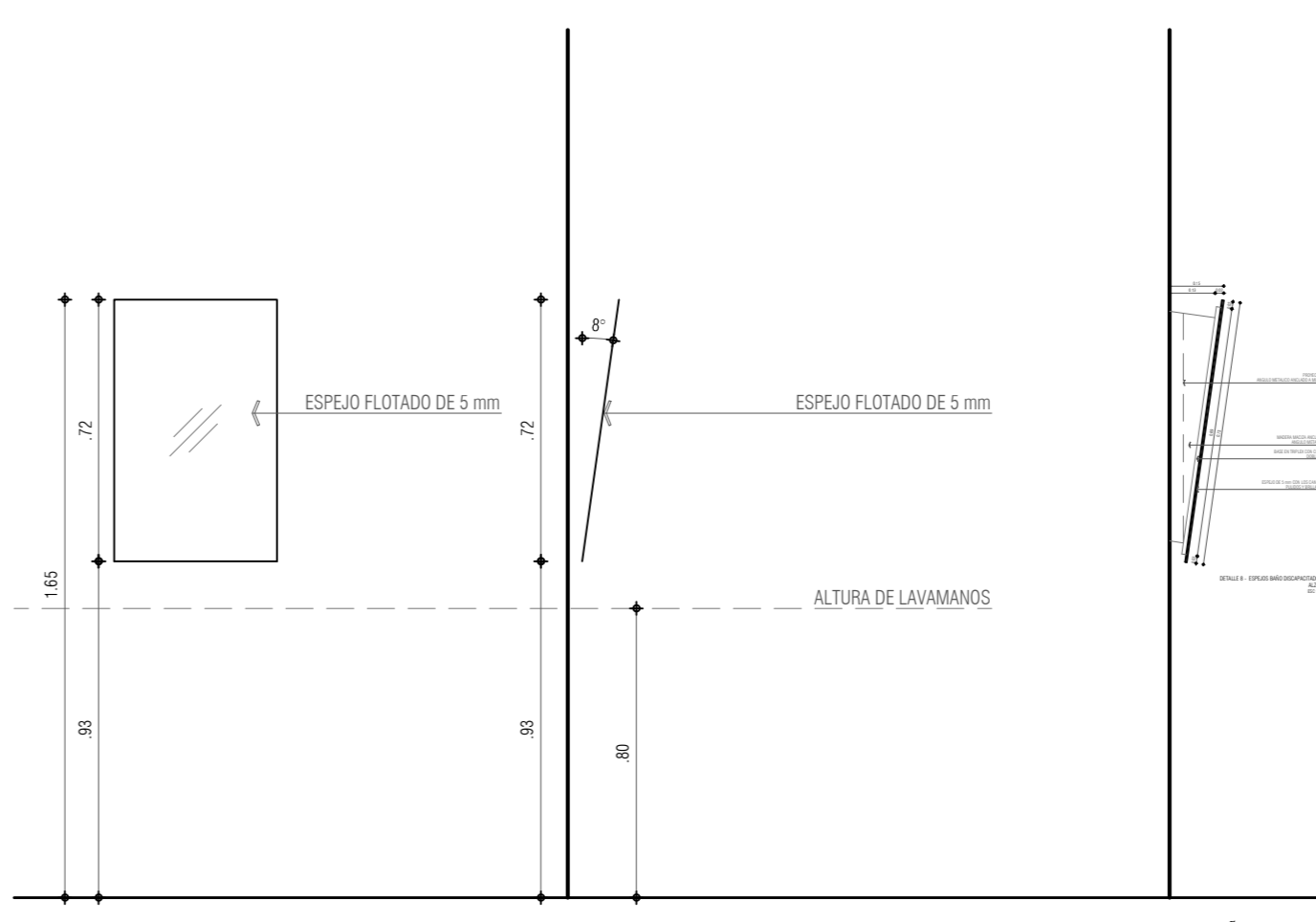
DETALLE 5 - ESPEJOS BAÑOS MOVILIDAD REDUCIDA ALZADO GENERAL - CORTE ESC 1_20
