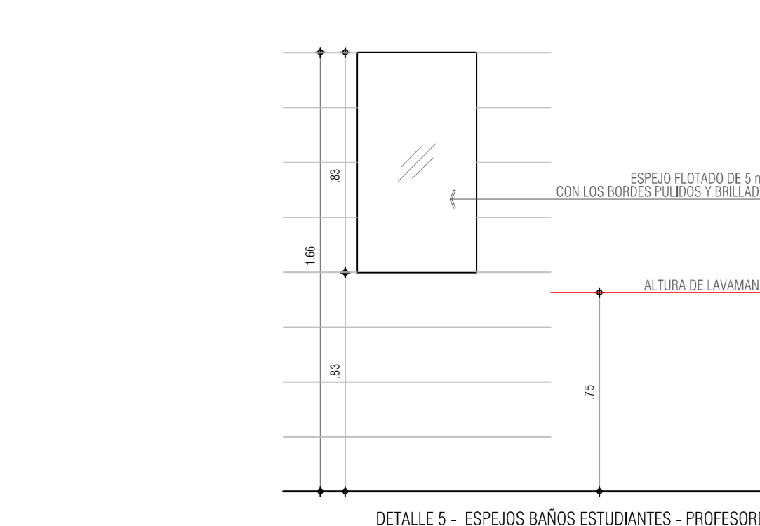
DETALLE 5 - ESPEJOS BAÑOS ESTUDIANTES - PROFESORES ALZADO GENERAL ESC 1_20
