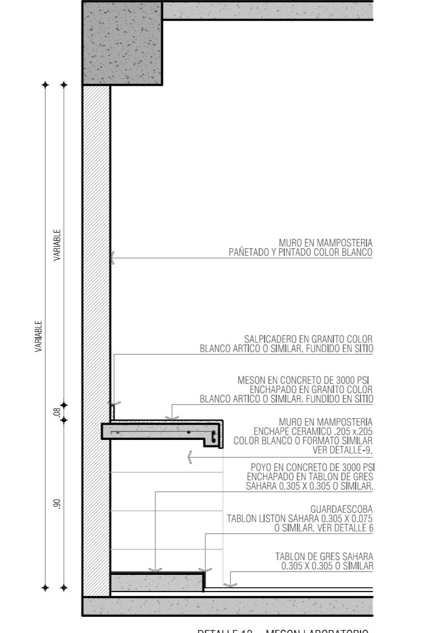
DETALLE 12 - MESÓN LABORATORIO ALZADO ESC 1_20
