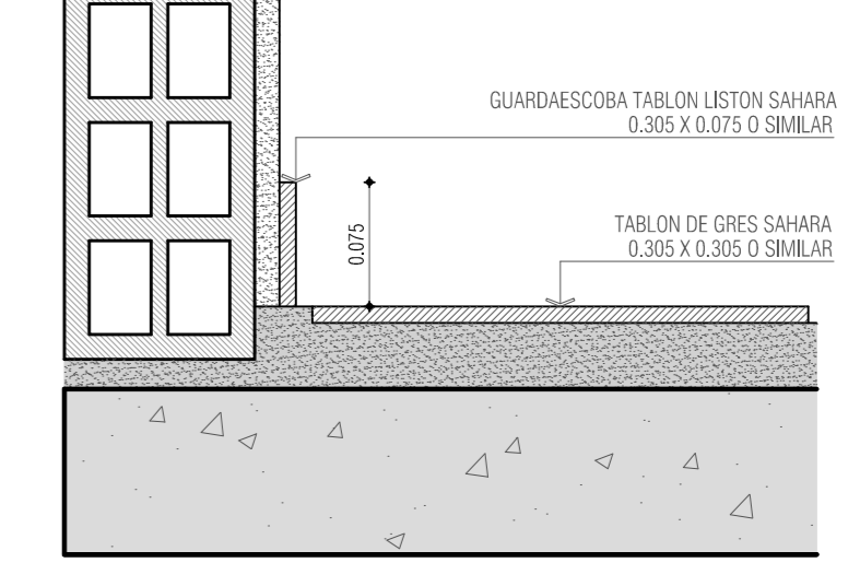
DETALLE 14 - GUARDAESCOBAS PISO EN TABLÓN DE GRES CORTE ESC 1_5
