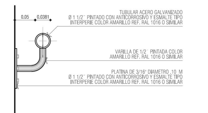
DETALLE 8 - PASAMANOS ESCALERA CORTE ESC 1_5
