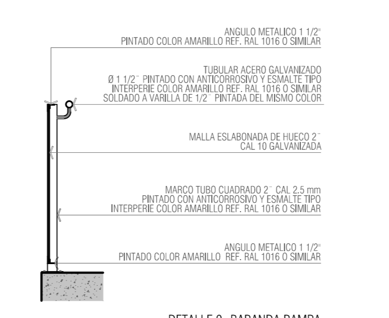
DETALLE 9 - BARANDA RAMPA CORTE ESC 1_50
