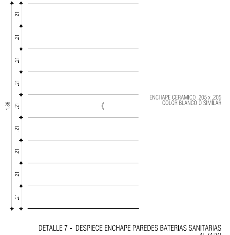
DETALLE 7 - DESPEQUE ENCHAFE PAREDES BATERIAS SANITARIAS ALZADO ESC 1_20
