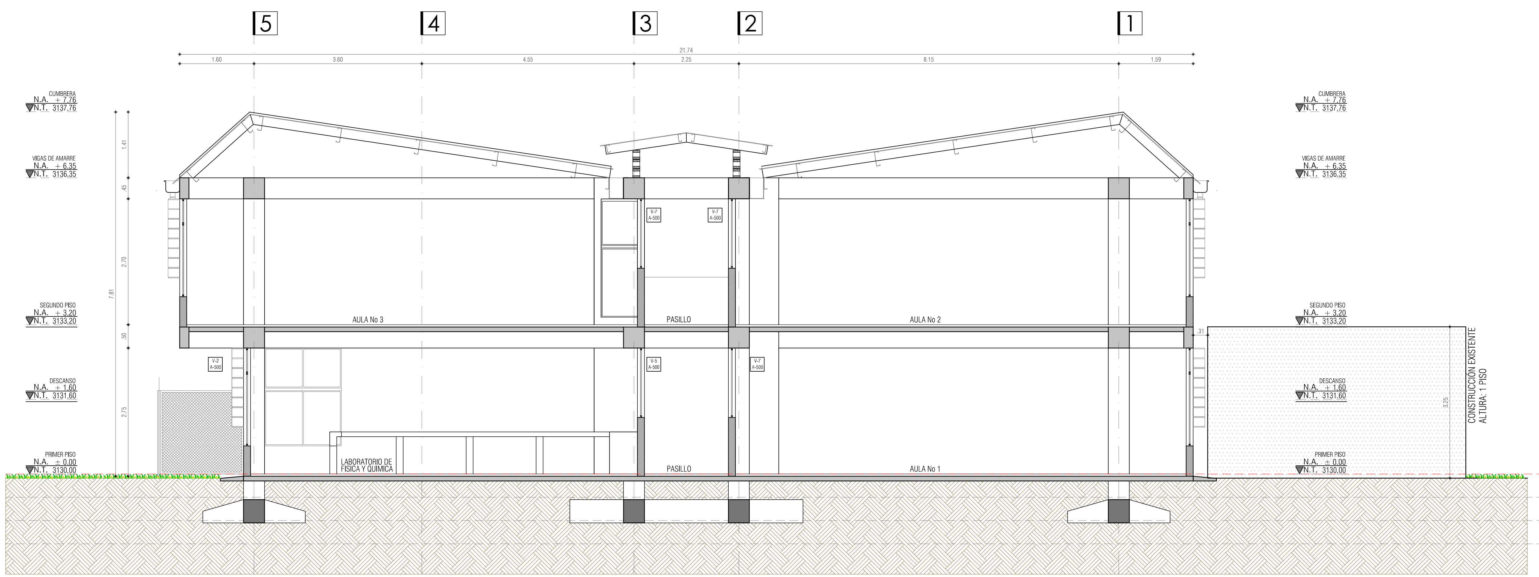
C.E.M EL SOCORRO BAJO CASANARE - PASTO CORTE GENERAL 1 ESC 1_50
