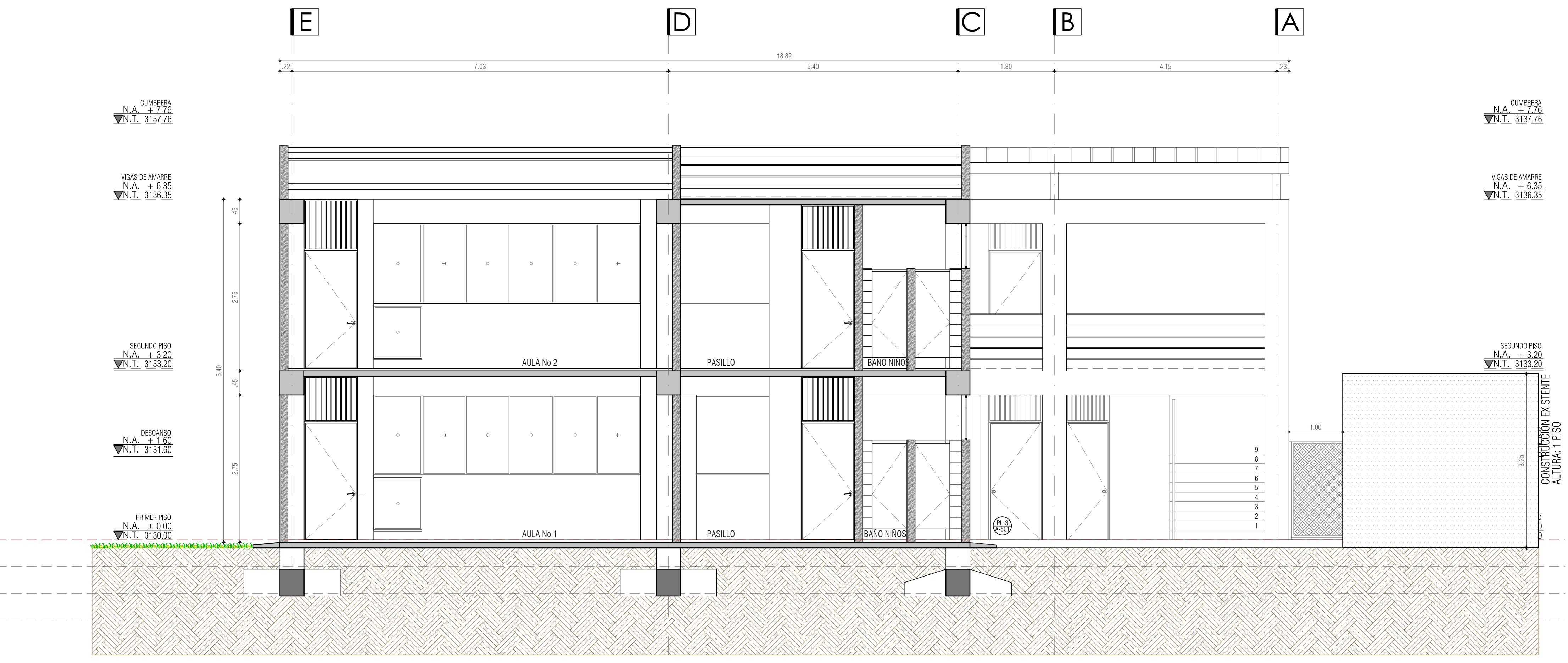
C.E.M EL SOCORRO BAJO CASANARE - PASTO CORTE GENERAL 2 ESC 1_50
