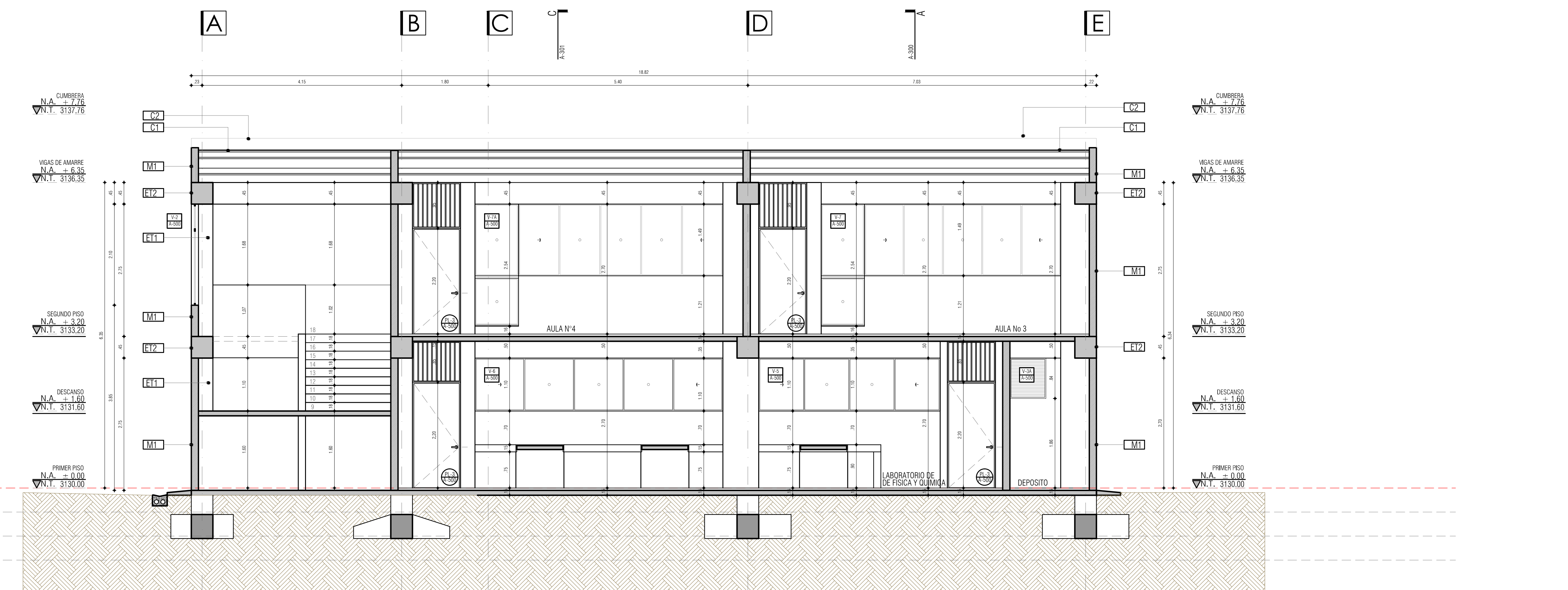
C.E.M EL SOCORRO BAJO CASANARE - PASTO CORTE C-C ESC 1_50
