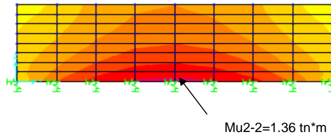
FIGURA 7. DIAGRAMA DE MOMENTO M2-2 (COMB 3) MURO 1
