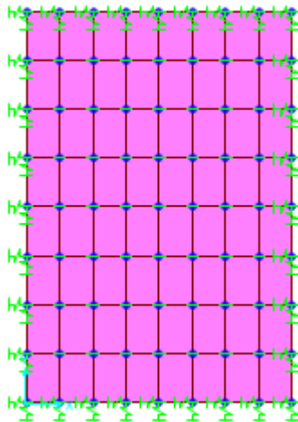
FIGURA 3. APOYO TANQUE DE ALMACENAMIENTO K_s = 1049 \text{ Ton/m}^3
