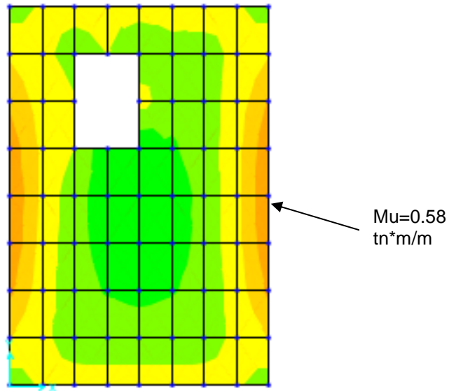
FIGURA 14. DIAGRAMA DE MOMENTO M1-1 – Losa Superior
