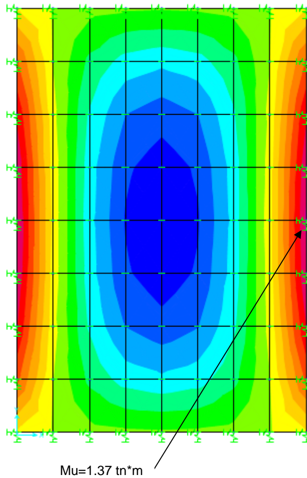
FIGURA 12. DIAGRAMA DE MOMENTO M1-1 – LOSA DE FONDO
