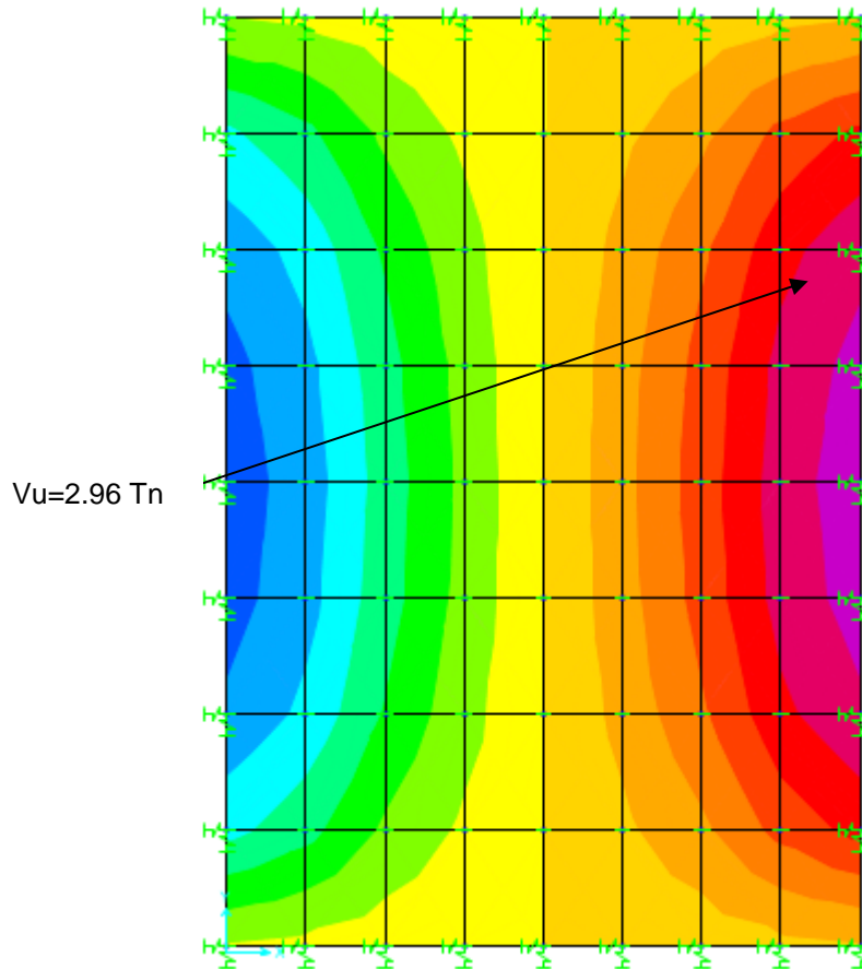
FIGURA 13. DIAGRAMA DE CORTANTE V1-3- LOSA DE FONDO
