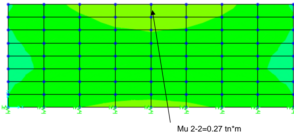
FIGURA 10. DIAGRAMA DE MOMENTO M2-2 (COMBO 3) MURO 2
