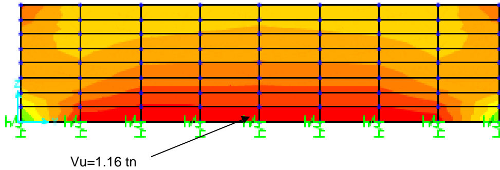
FIGURA 9. DIAGRAMA DE CORTANTE V23 – MURO 1
