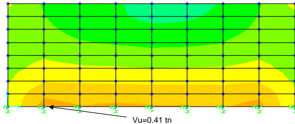
FIGURA 11. DIAGRAMA DE CORTANTE V23 (COMBO 3) MURO 2
