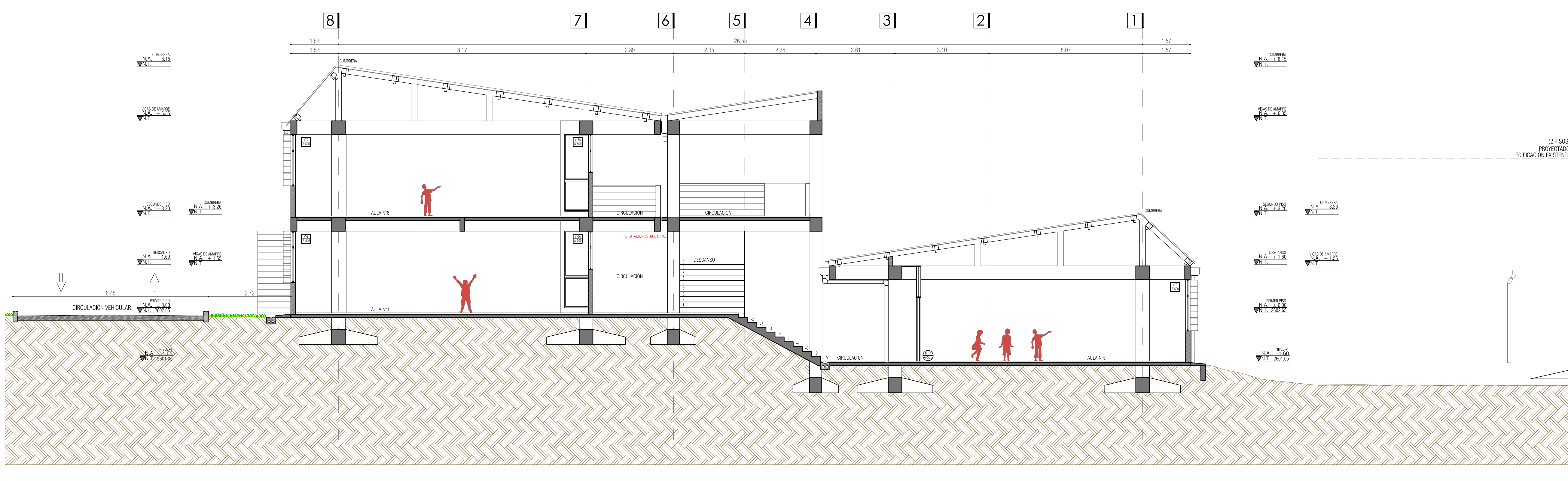
I.E. INEM - PASTO CORTE GENERAL 2 ESC 1_75
