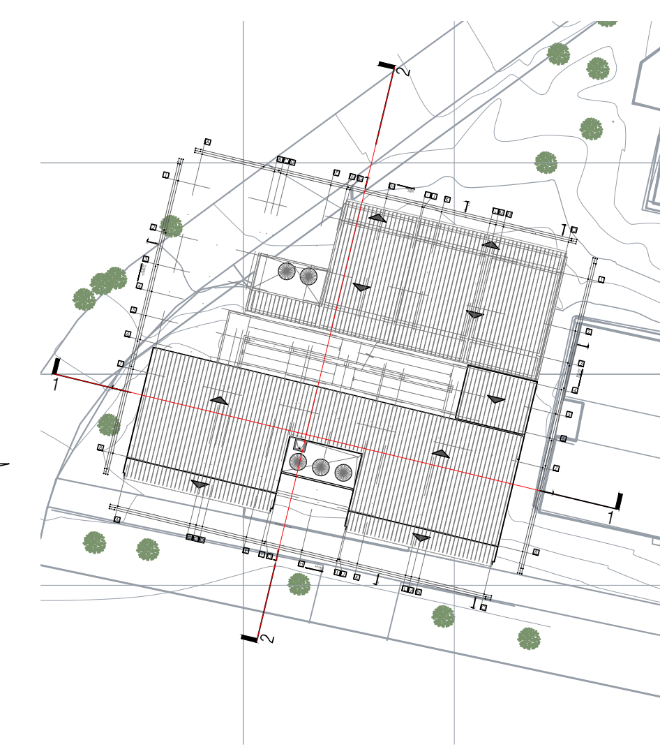
I.E. INEM - PASTO LOCALIZACION ESC 1_800
