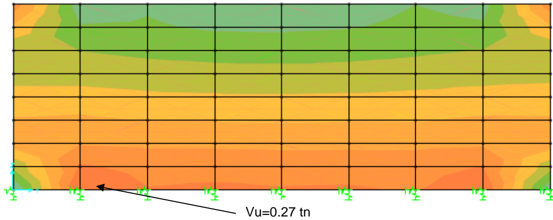
FIGURA 9. DIAGRAMA DE CORTANTE V23 – MURO 1
