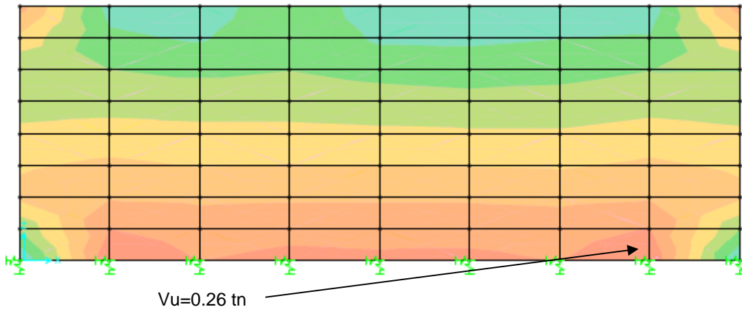
FIGURA 11. DIAGRAMA DE CORTANTE V23 (COMBO 3) MURO 2
