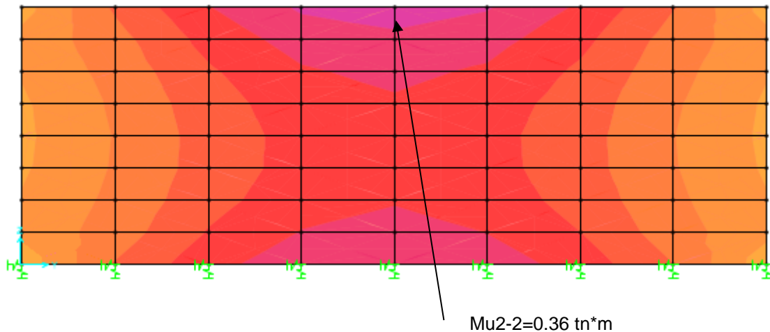
FIGURA 7. DIAGRAMA DE MOMENTO M2-2 (COMB 3) MURO 1
