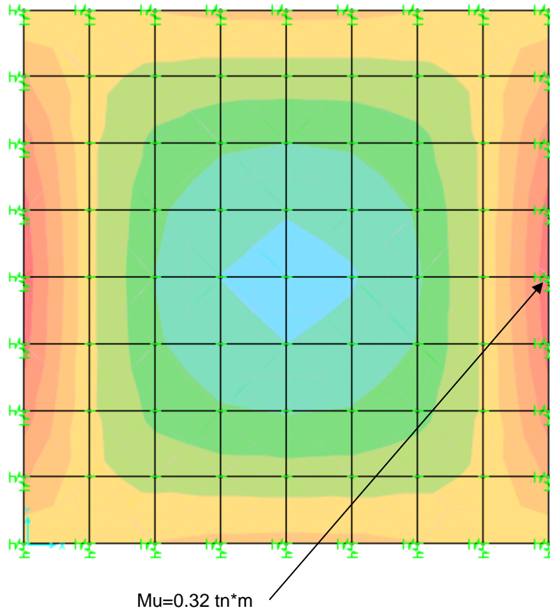
FIGURA 12. DIAGRAMA DE MOMENTO M1-1 – LOSA DE FONDO
