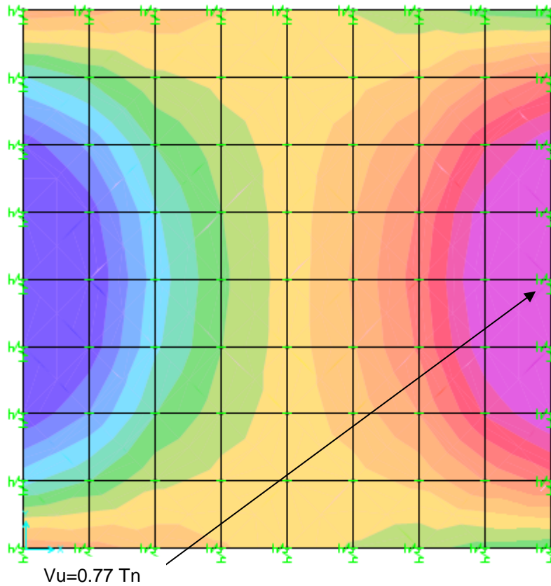
FIGURA 13. DIAGRAMA DE CORTANTE V1-3- LOSA DE FONDO
