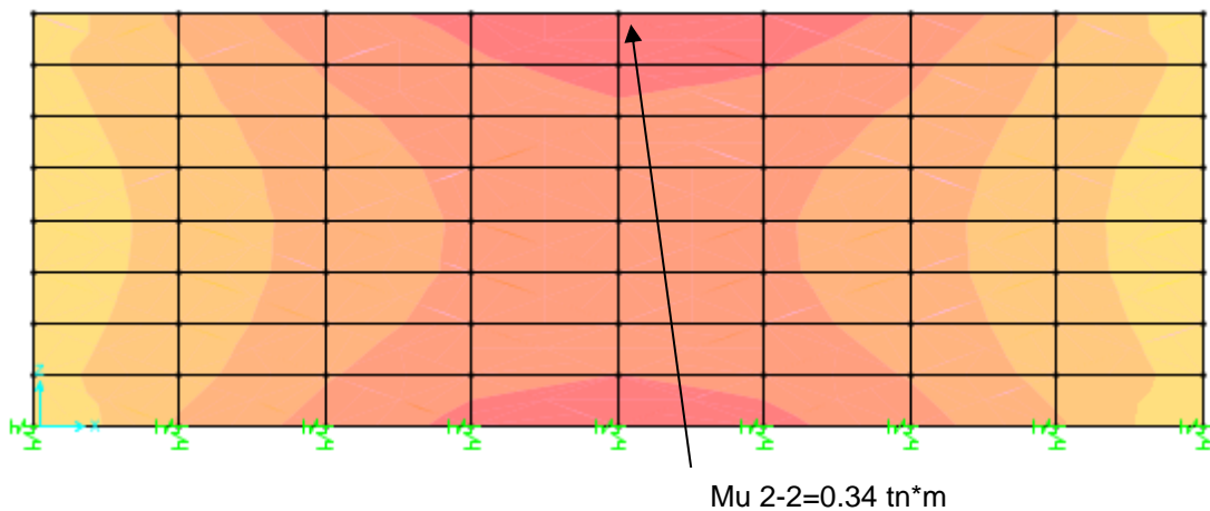
FIGURA 10. DIAGRAMA DE MOMENTO M2-2 (COMBO 3) MURO 2
