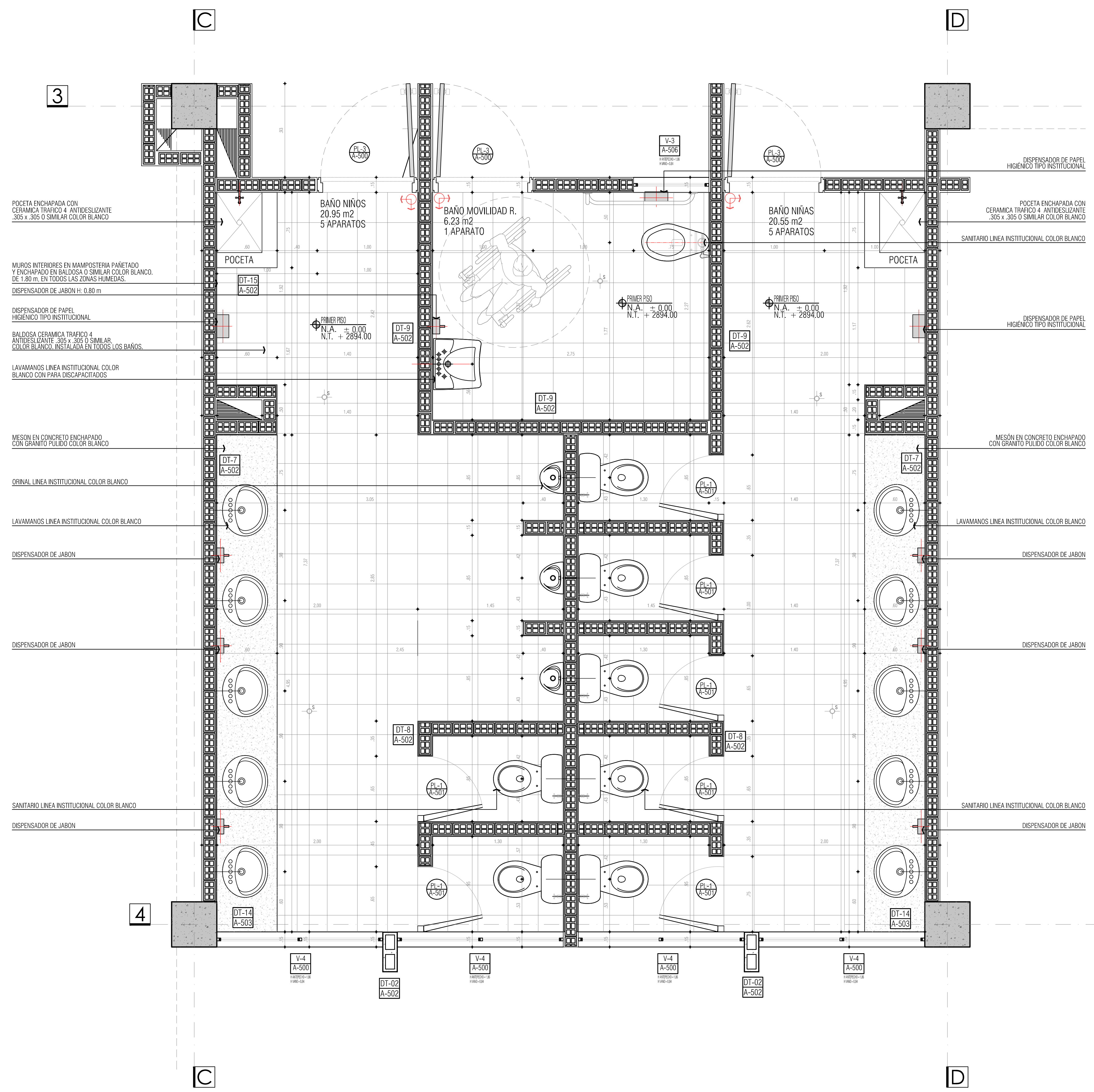
LE SEMINARIO - IPIALES DETALLE BATERIA SANITARIA PISO 1 - PISO 2 ESC 1_20
