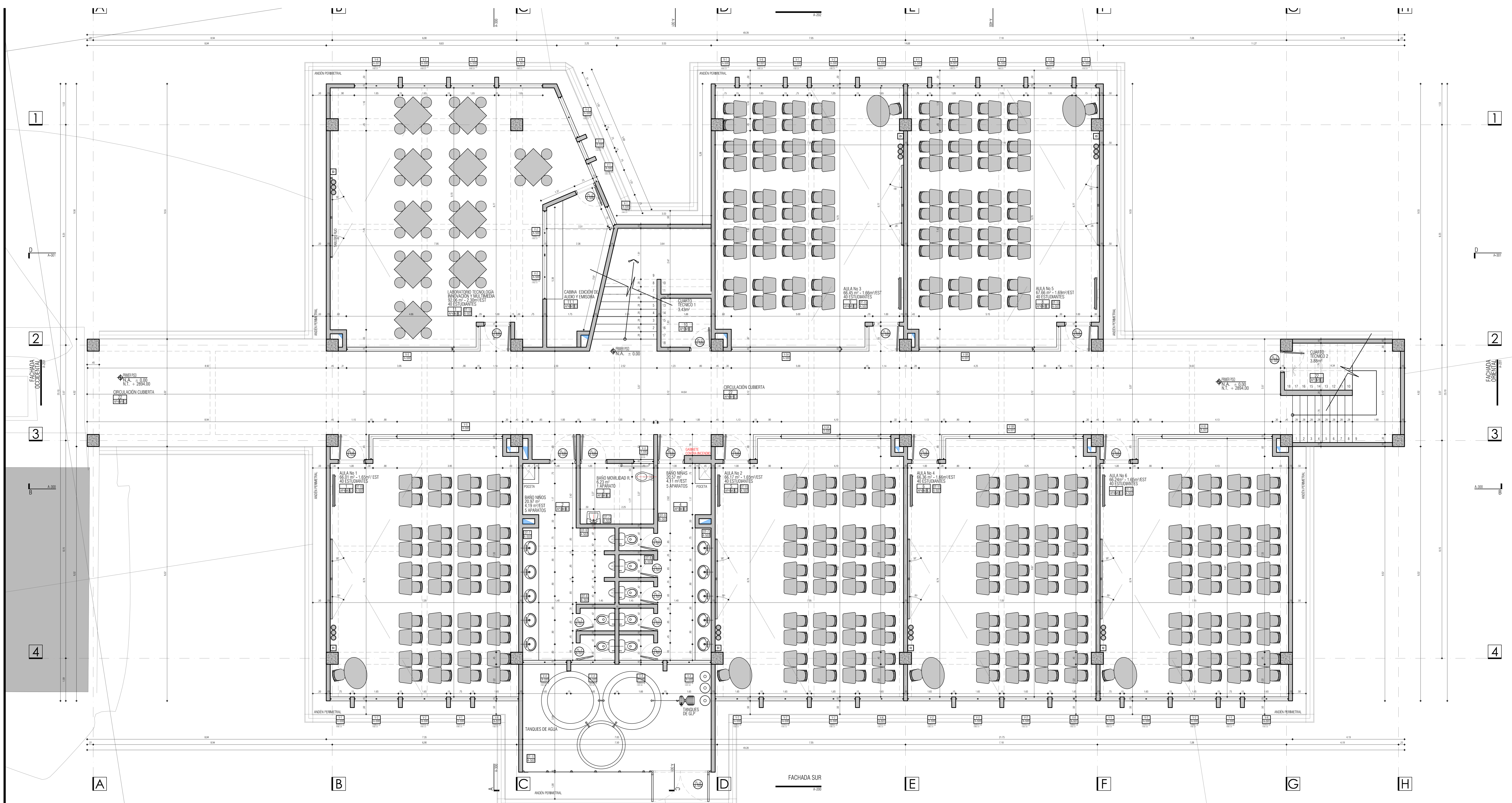
I.E. SEMINARIO - IPIALES PLANTA PRIMER PISO ESC 1:50
