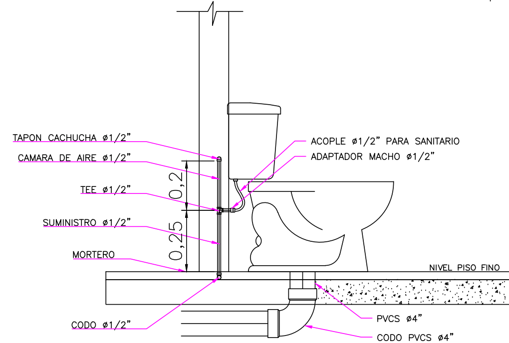
DETALLE MONTAJE INODORO Sin Escala
