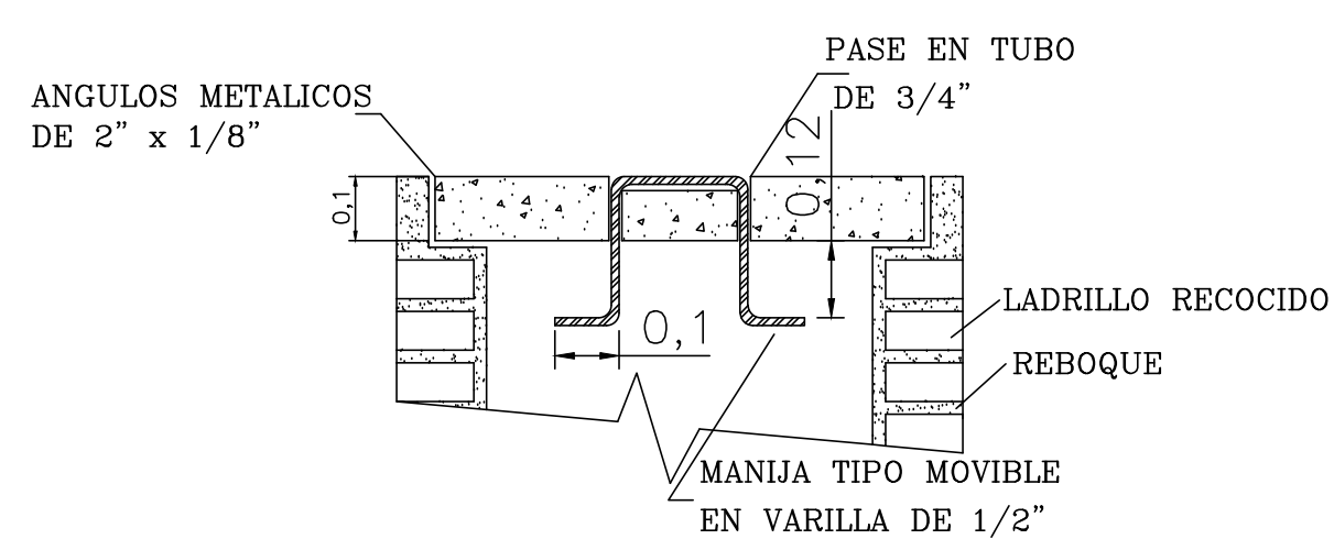
TAPA CAJA DE INSPECCION
