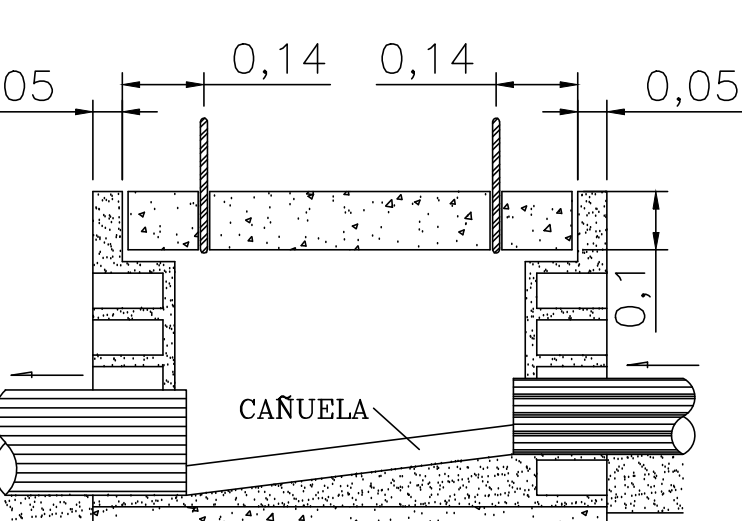
CONCRETO PLACA DE CONCRETO REFORZADO CON HIERRO DE 3/8 RECEO COMPACTADO
