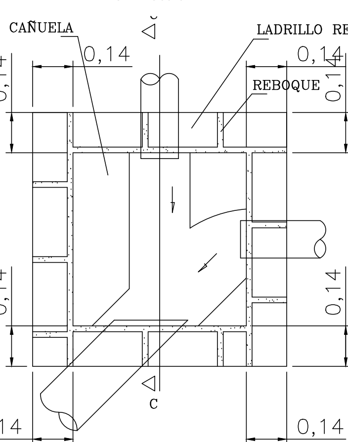
DETALLE MONTAJE INODORO INFANTIL Sin Escala
