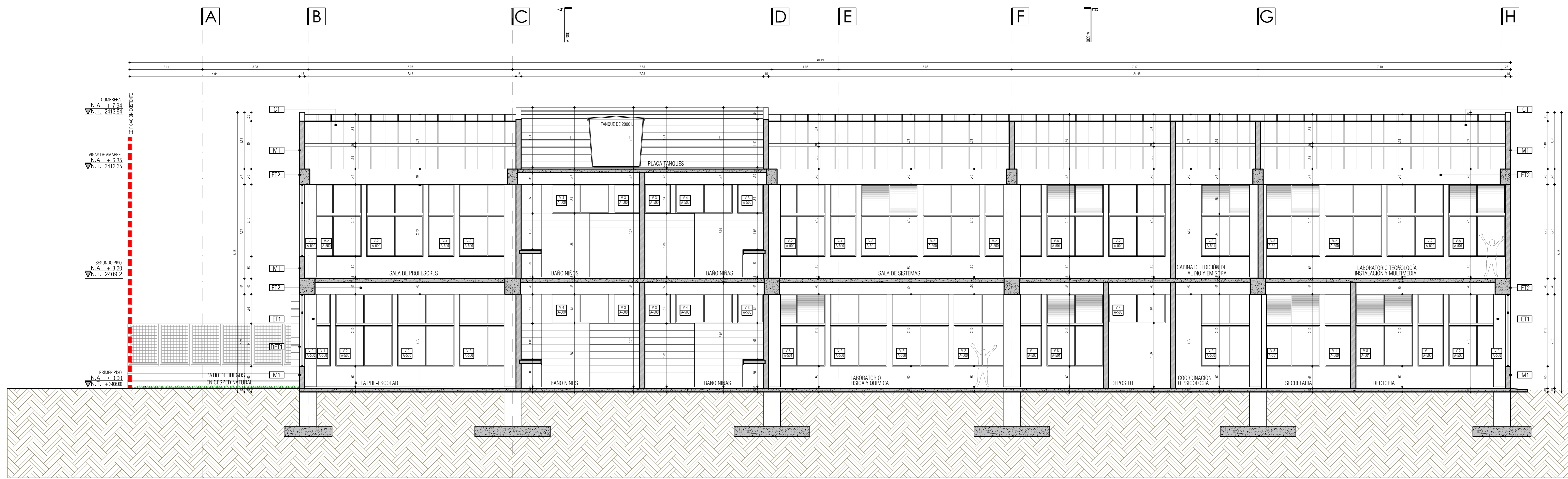
I.E. SAN JUAN - IPIALES CORTE C-C ESC 1 - 50
