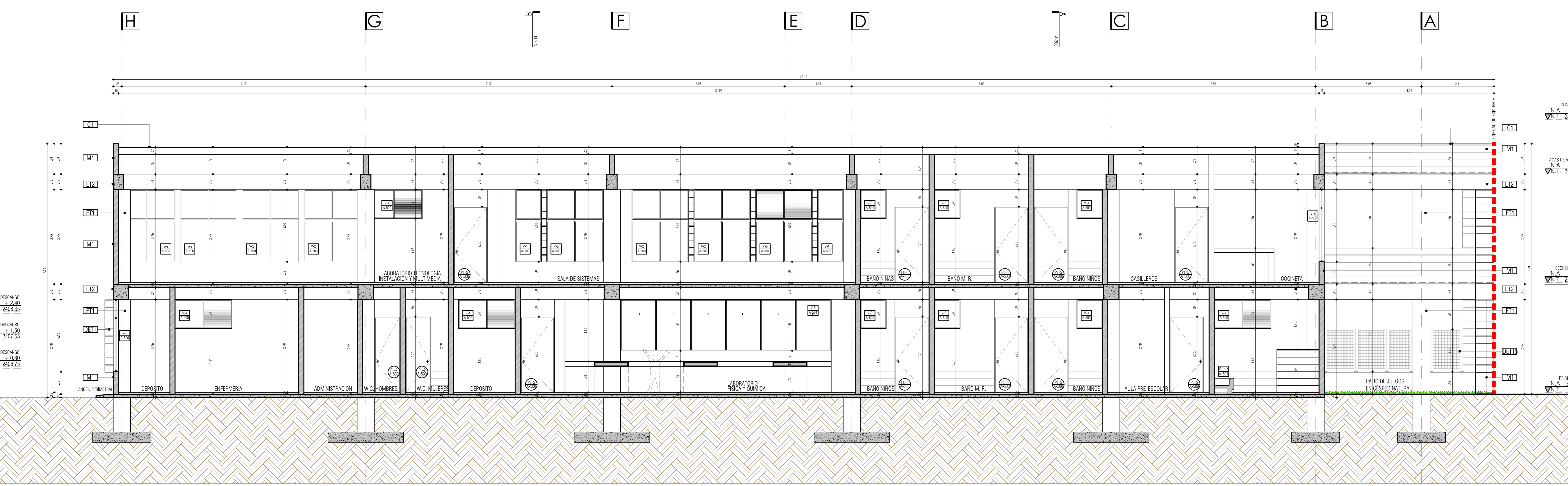
I.E. SAN JUAN - IPIALES CORTE D-D ESC 1 - 50
