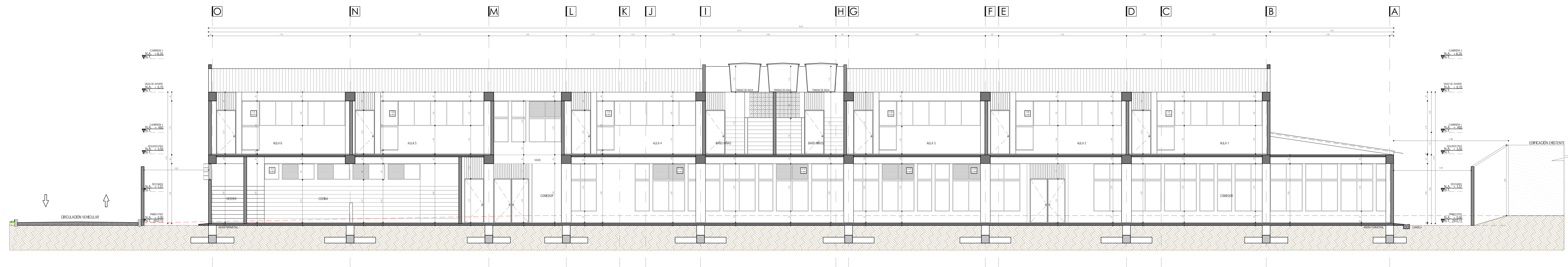
I.E. POLITECNICO MARCELO MIRANDA CORTE GENERAL 1 ESC. 1_75
