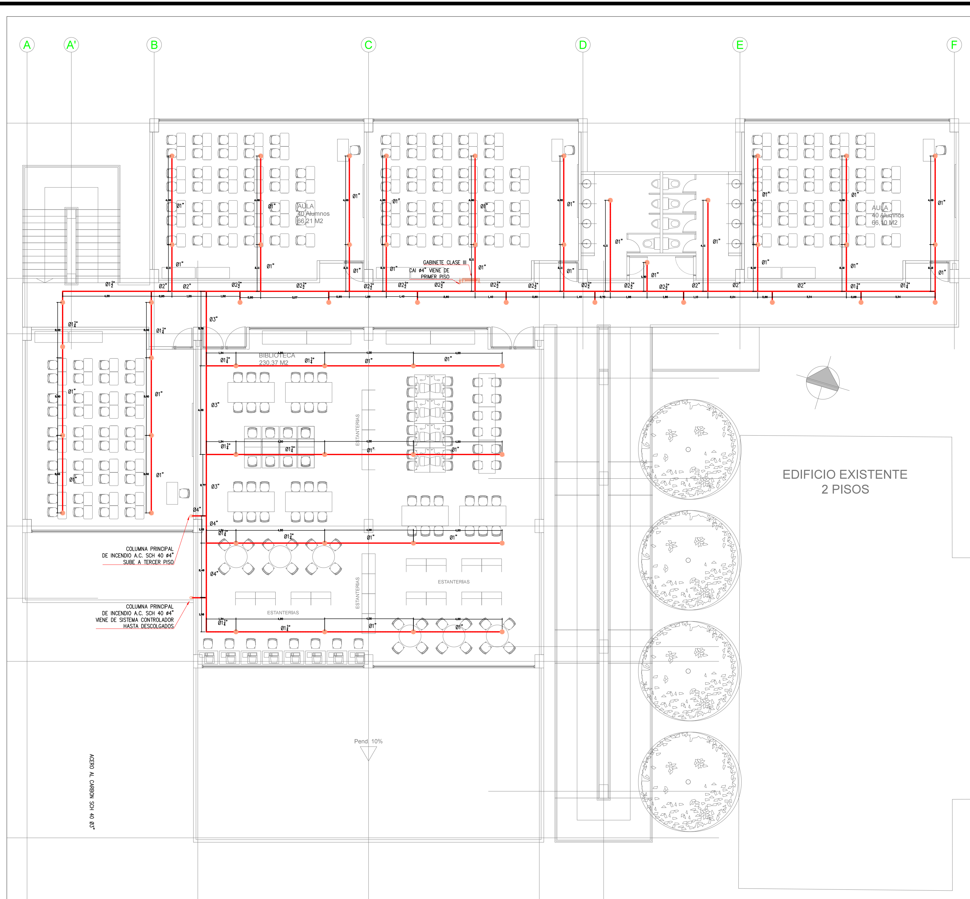
RED CONTRA INCENDIO PLANTA SEGUNDO ESCALA 1:100
