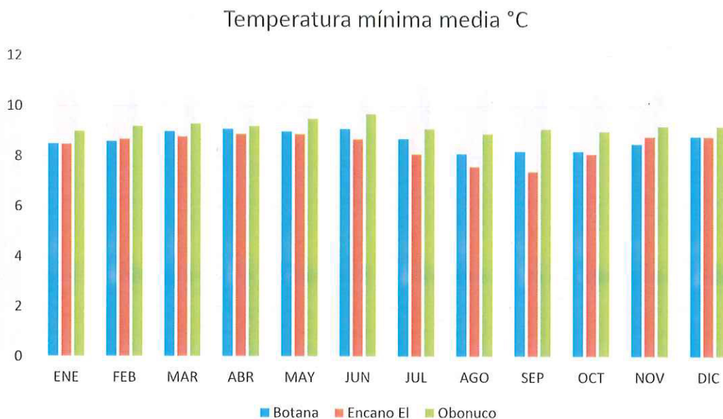
Grafico 4-2 Temperatura mínima media
