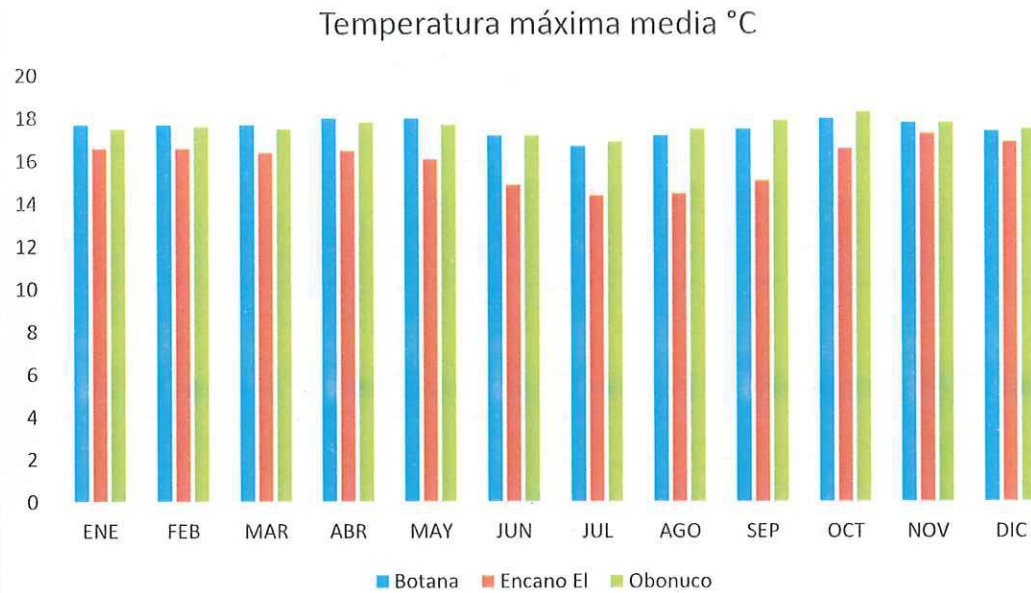
Grafico 4-1 Temperatura máxima media
