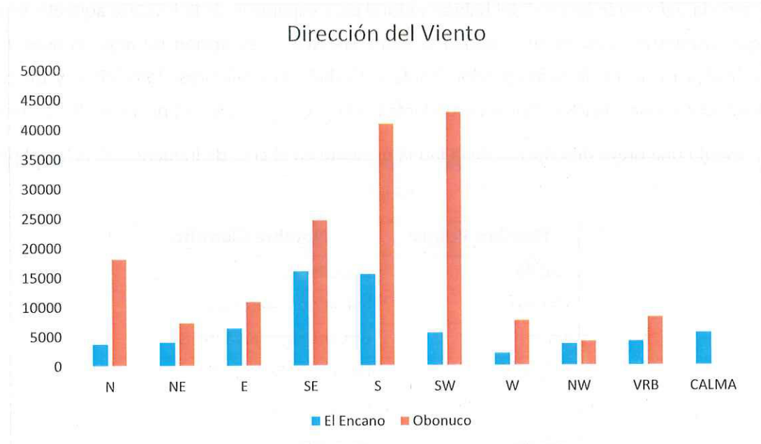
Gráfico 4-8 Dirección del Viento
