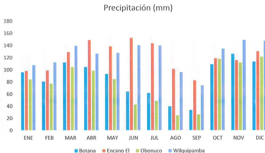
Grafico 4-3 Promedio de Precipitación
