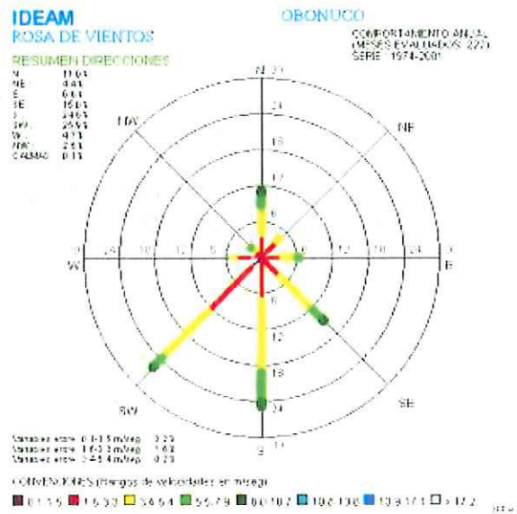
Grafico 4-7 Rosas de los Vientos
