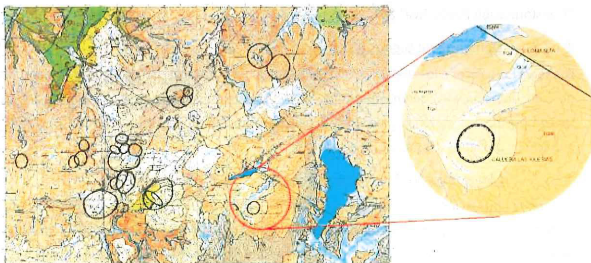
Ilustración 4-1 Mapa Geológico Plancha 429 Pasto
