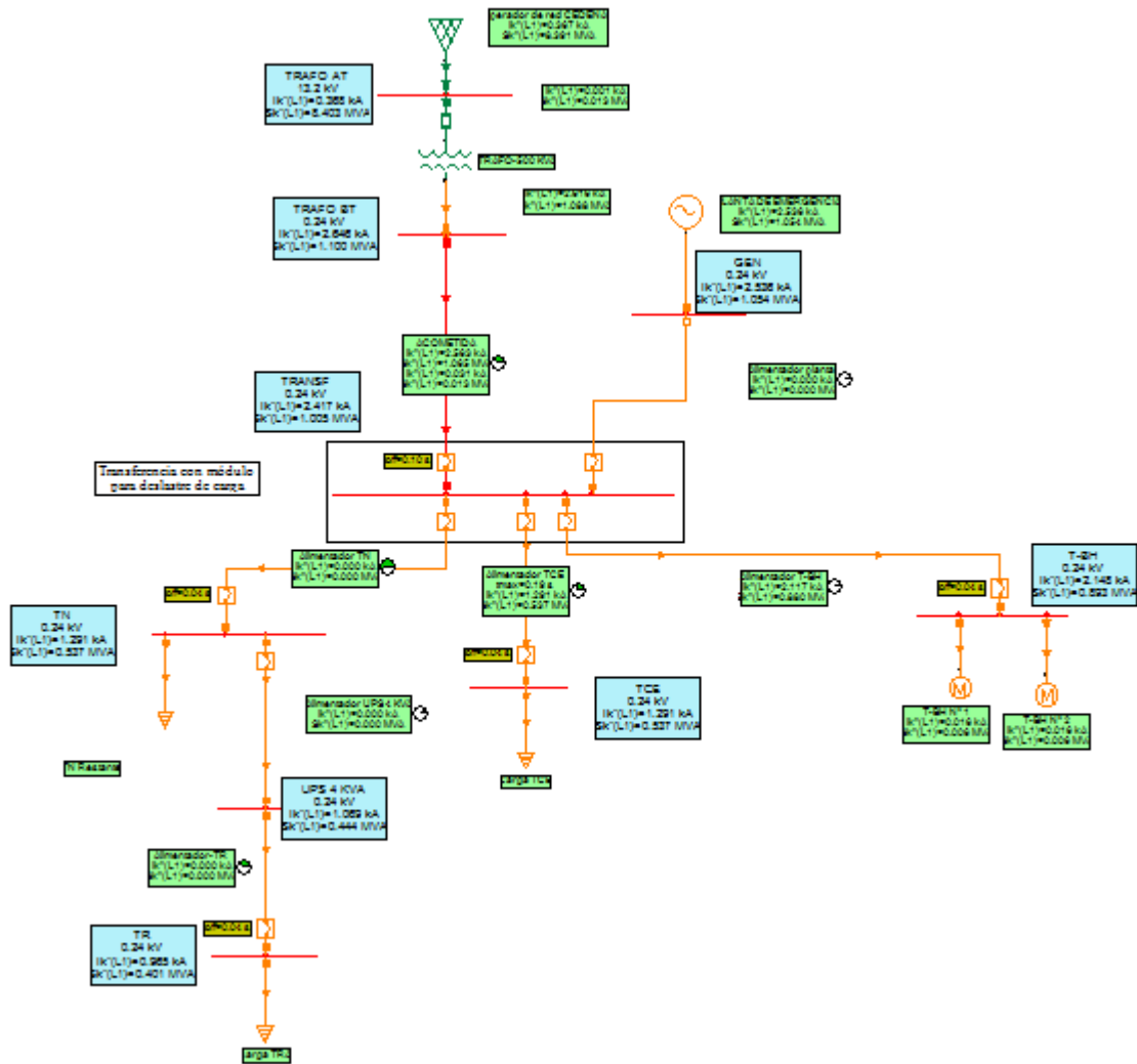
Figura 5 Análisis de corto circuito en NEPLAN
