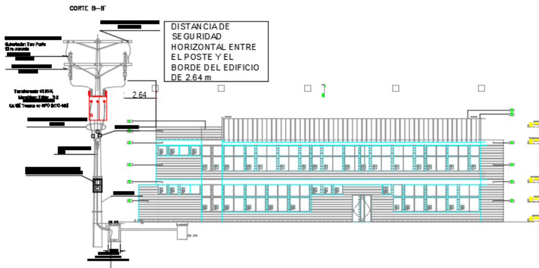
Figura 7 Corte de subestación para evidenciar distancia de seguridad
