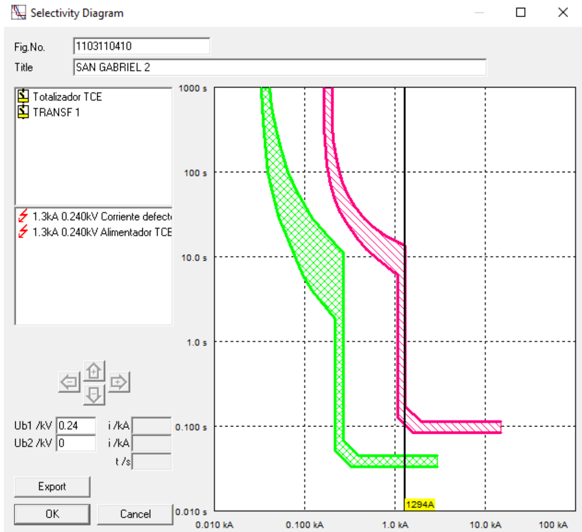
Grafica 3 Coordinación de la protección del tablero general de acometida y protección de red normal de transferencia
