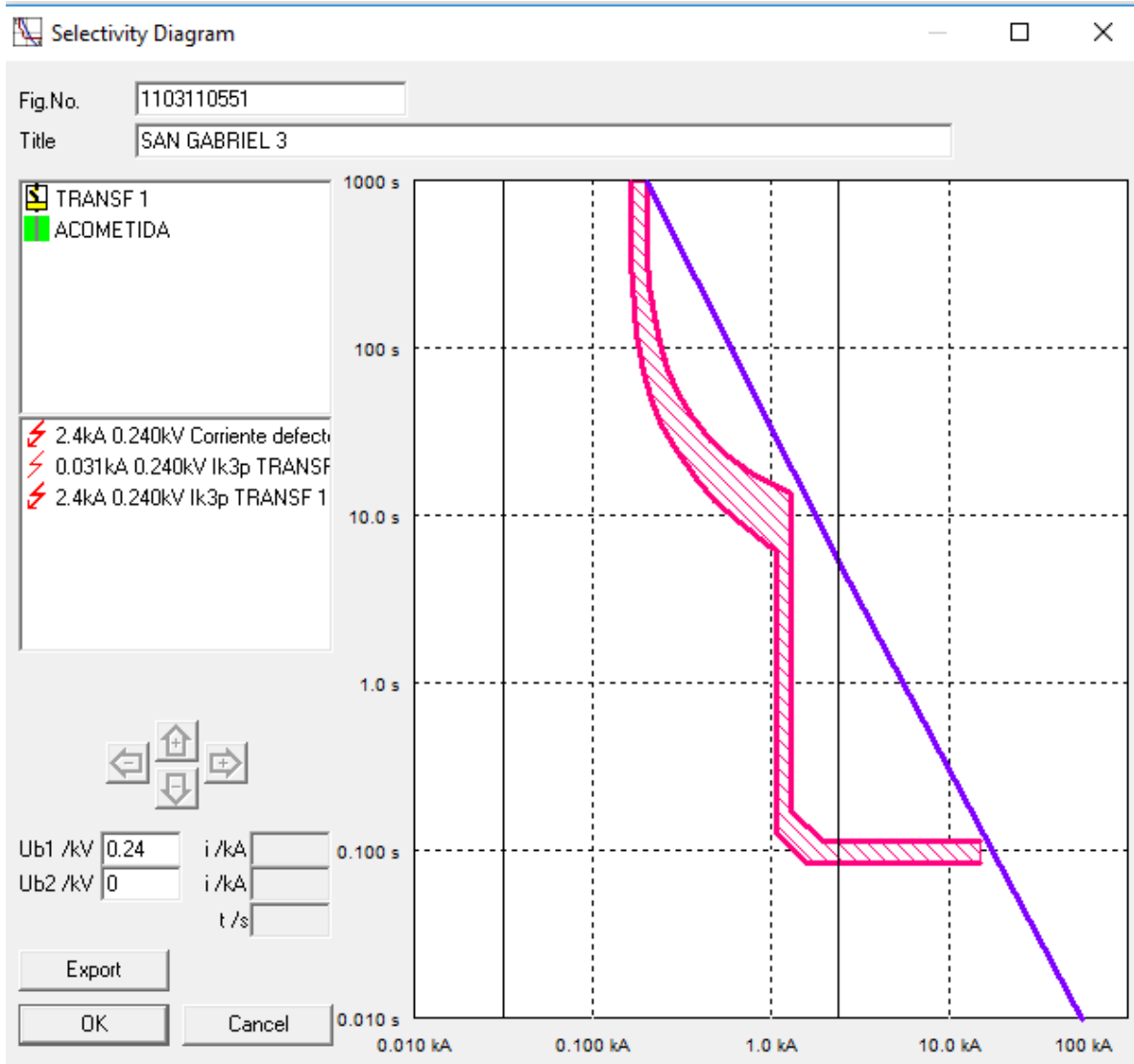
Grafica 4 Grafica de coordinación de la protección en el barraje de la transferencia
