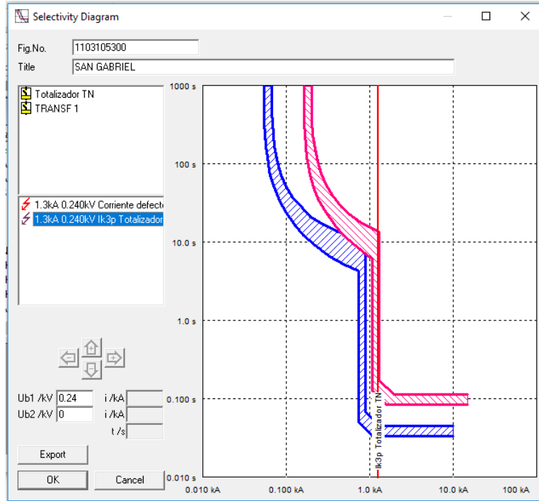
Grafica 2 Coordinación de la protección del tablero normal del primer piso y protección de red normal de transferencia
