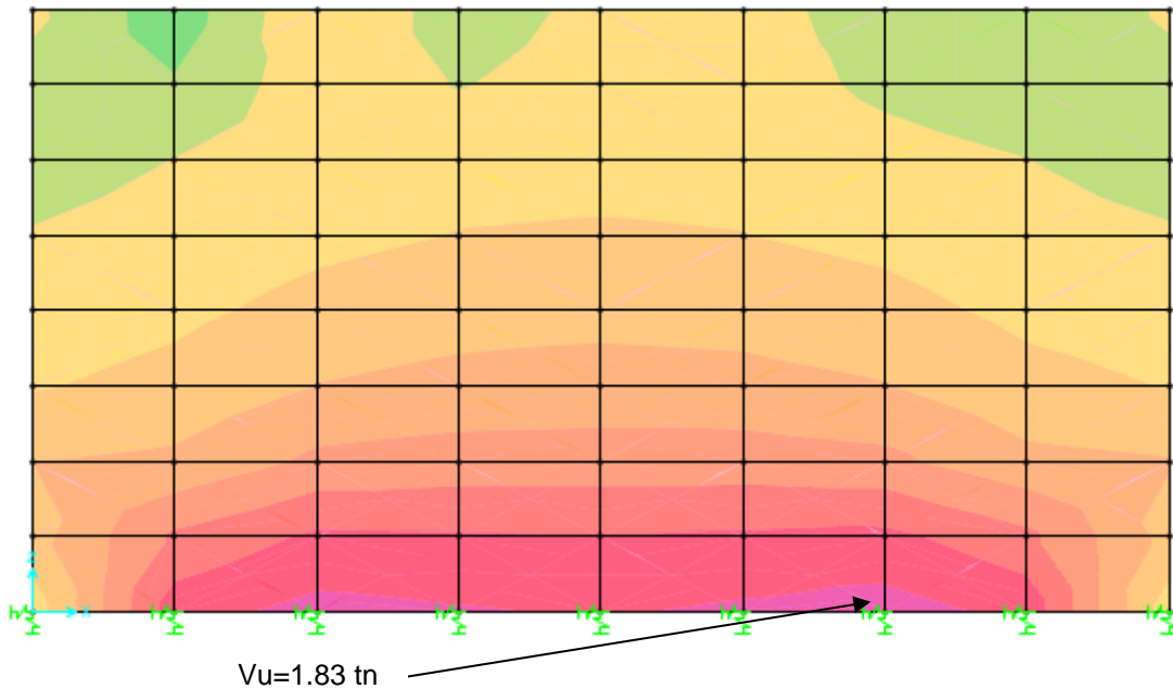
FIGURA 11. DIAGRAMA DE CORTANTE V23 (COMBO 3) MURO 2
