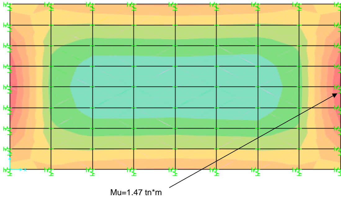
FIGURA 12. DIAGRAMA DE MOMENTO M1-1 – LOSA DE FONDO
