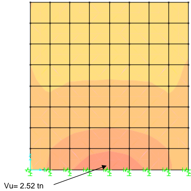
FIGURA 9. DIAGRAMA DE CORTANTE V23 – MURO 1
