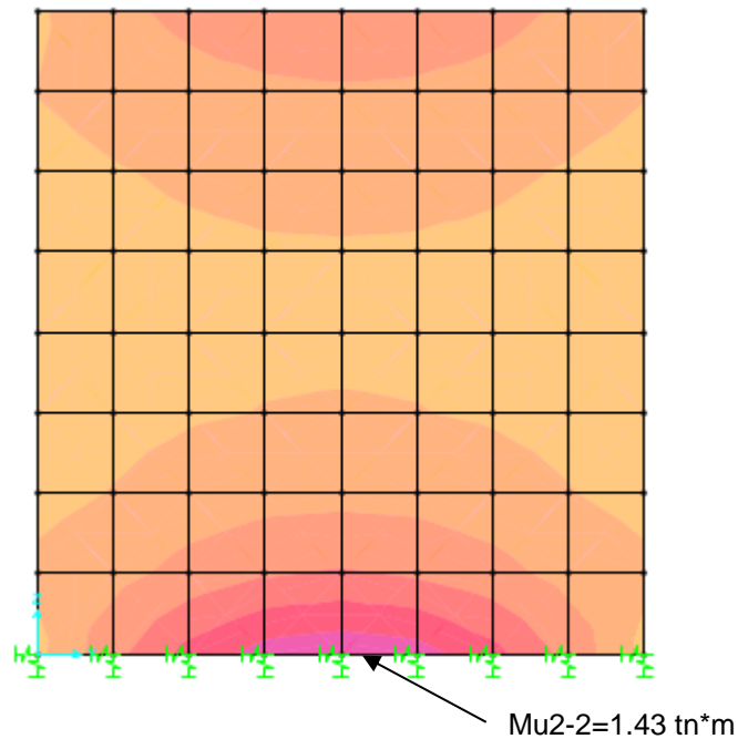
FIGURA 7. DIAGRAMA DE MOMENTO M2-2 (COMB 3) MURO 1
