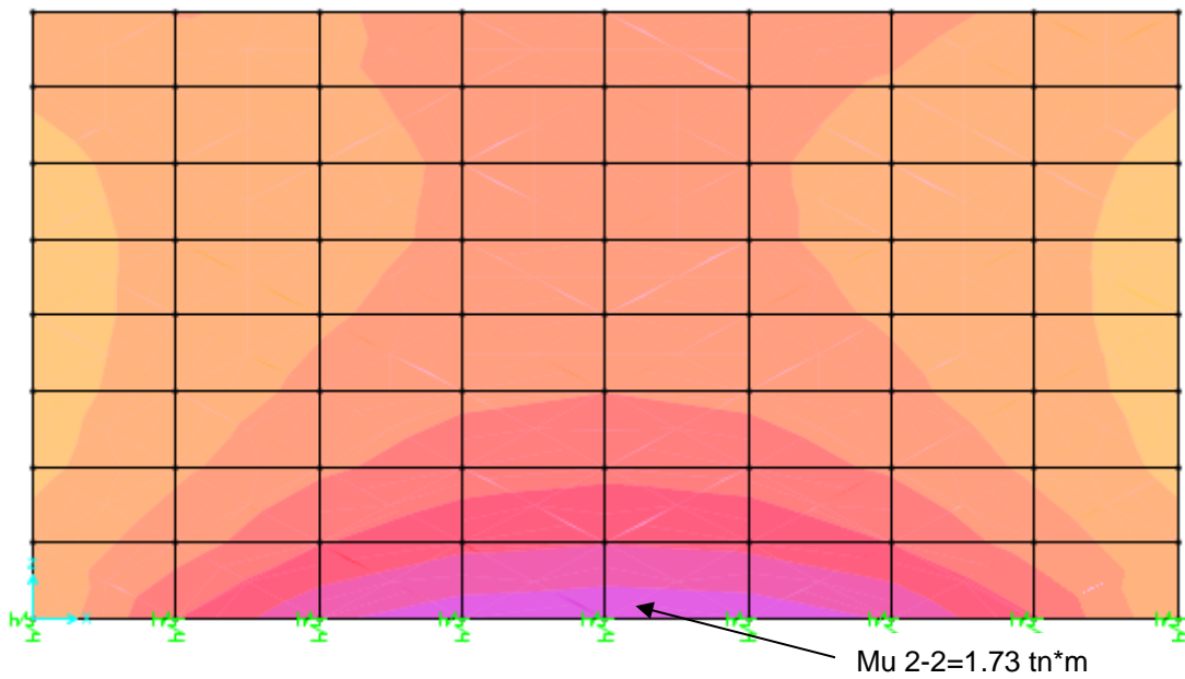
FIGURA 10. DIAGRAMA DE MOMENTO M2-2 (COMBO 3) MURO 2
