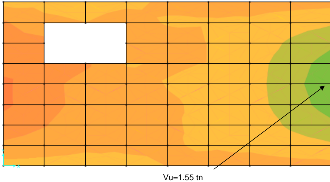
FIGURA 15. DIAGRAMA DE CORTANTE V13– Losa Superior
