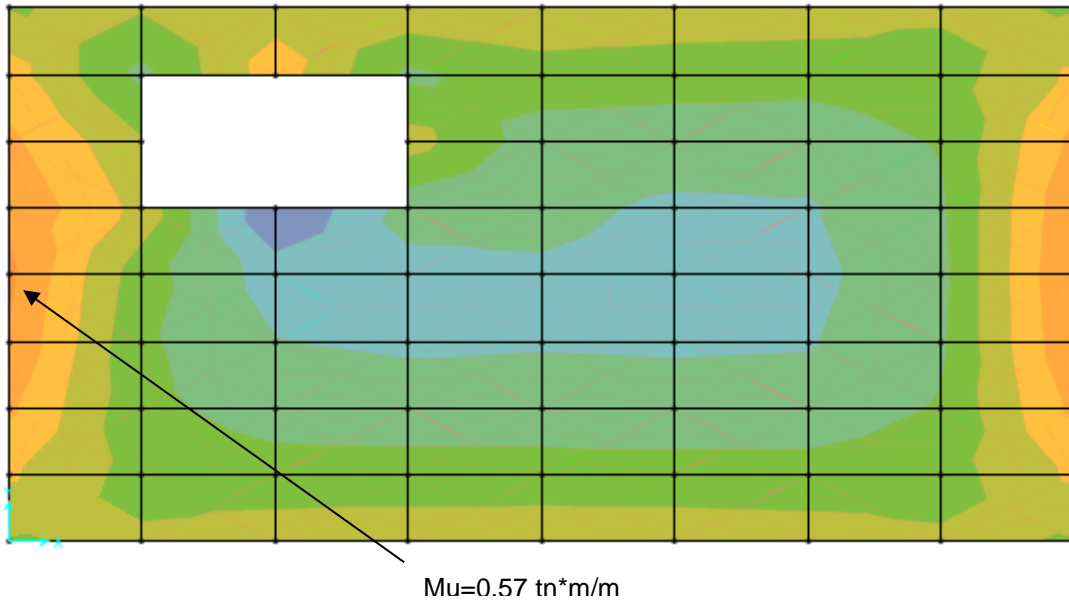
FIGURA 14. DIAGRAMA DE MOMENTO M1-1 – Losa Superior
