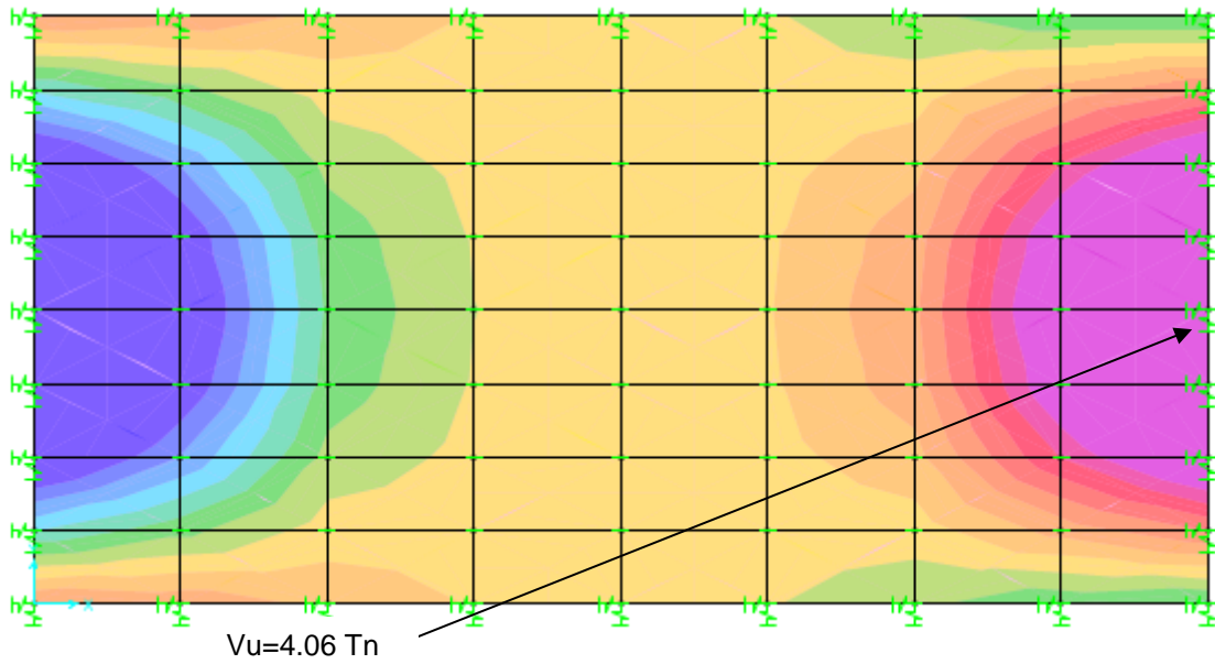
FIGURA 13. DIAGRAMA DE CORTANTE V1-3- LOSA DE FONDO
