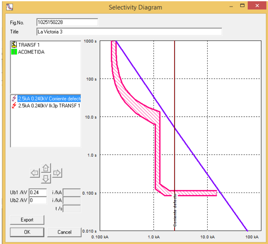
Grafica 4 Coordinación de la protección en el barraje y la curva de daño de la acometida principal.
