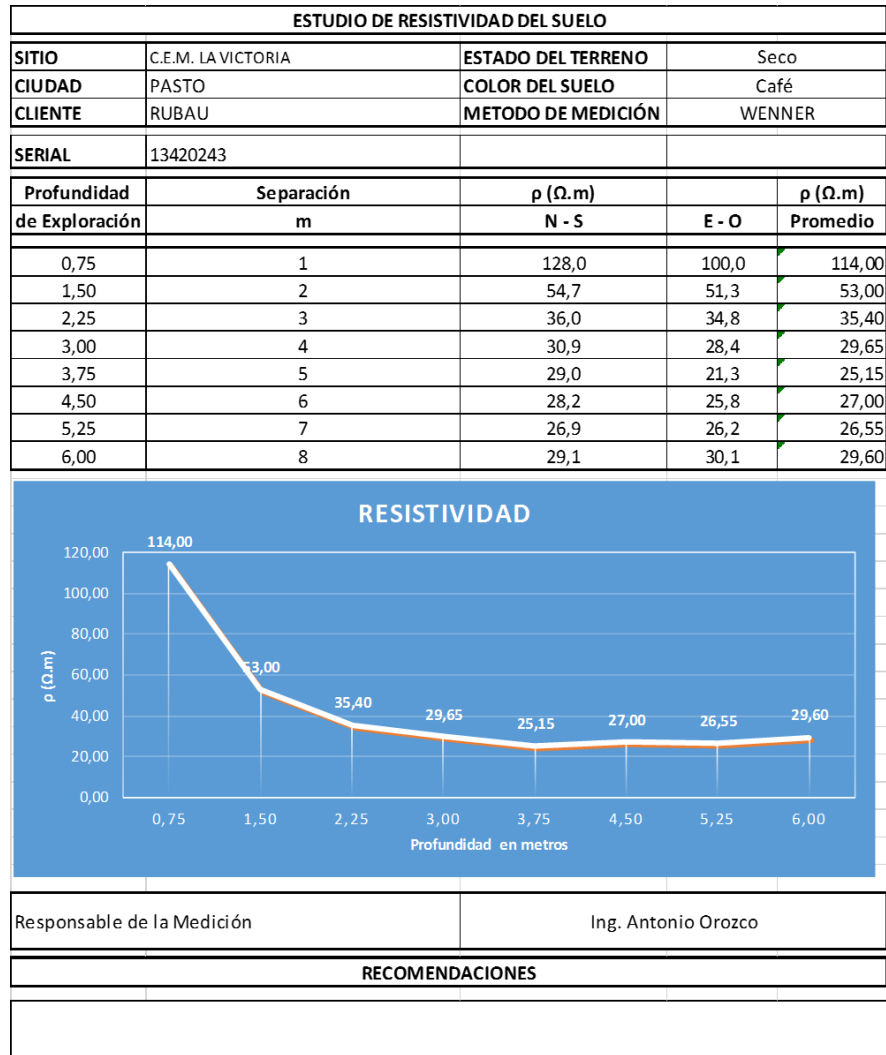
Grafica 5 Resultados de análisis de resistividad del terreno
