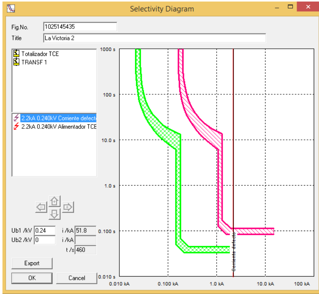
Grafica 3 Coordinación de la protección del tablero de circuitos esenciales y protección de red normal de transferencia
