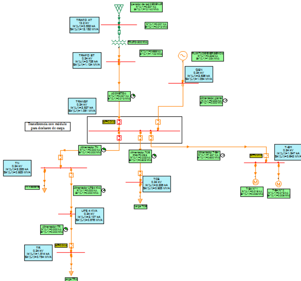
Figura 5 Análisis de corto circuito en NEPLAN
