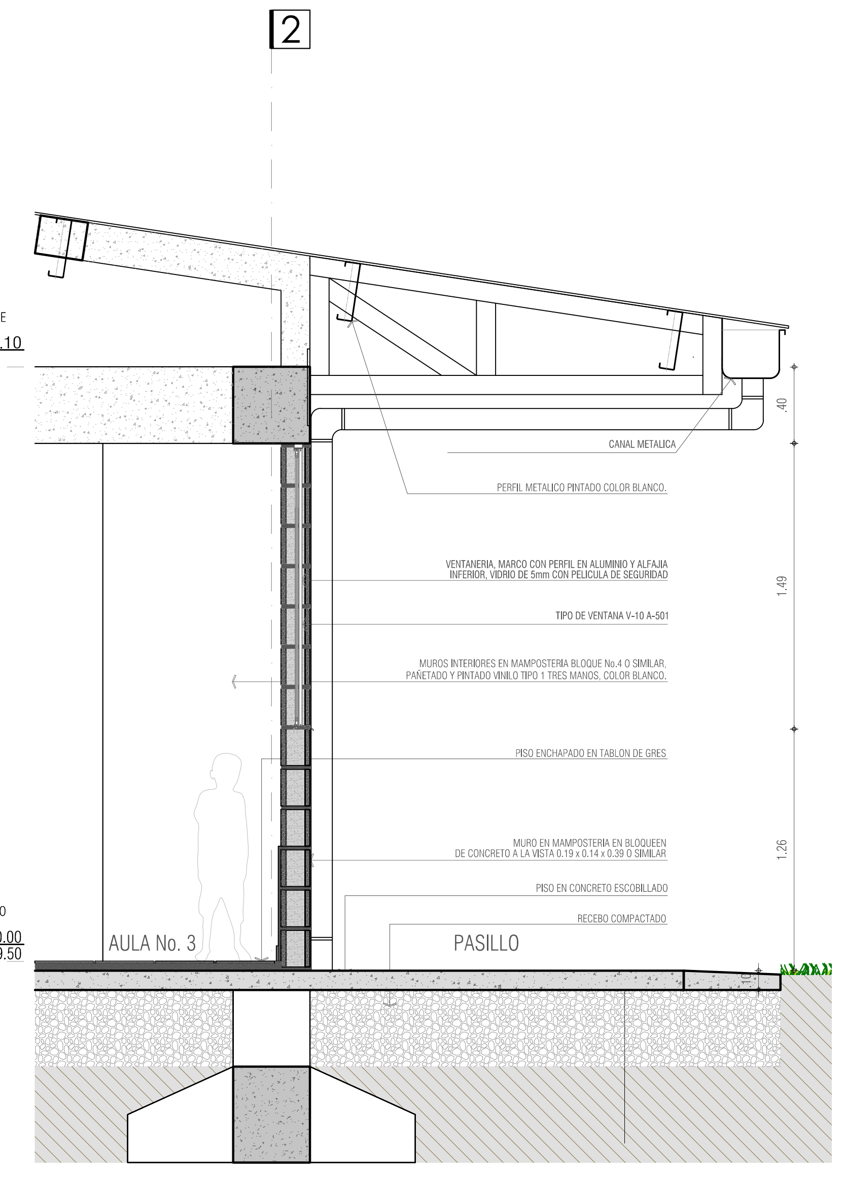
C.E.M. LA VICTORIA PASTO CORTE FACHADA 2 ESC 1_20
