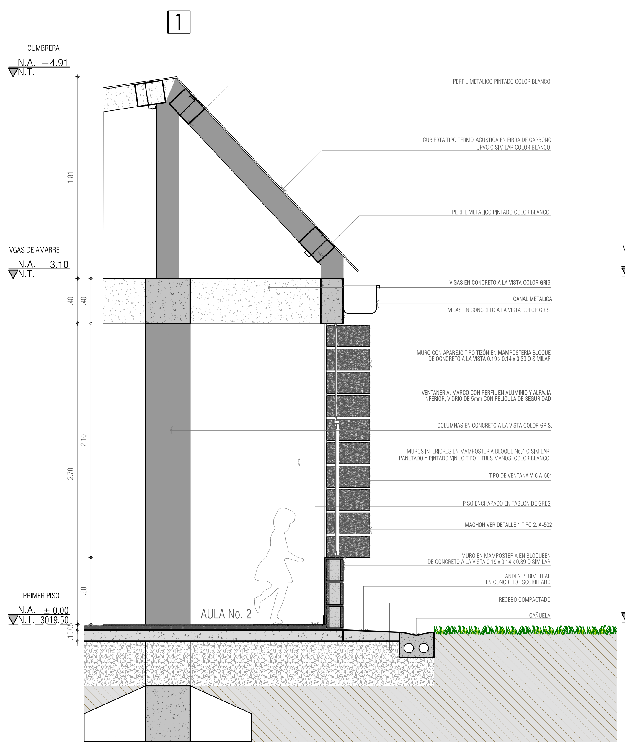
C.E.M. LA VICTORIA PASTO CORTE FACHADA 1 ESC 1_20
