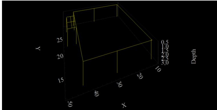
Figura 11 Puesta a tierra configuración cuadrada de 5x5 m interconectada con la red de protección contra rayos
