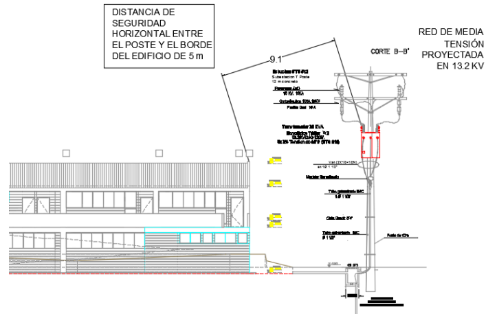
Figura 7 Corte de subestación para evidenciar distancia de seguridad
