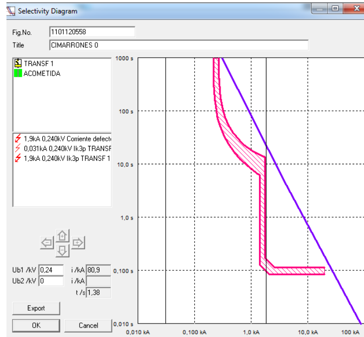
Grafica 5 Coordinación de la protección en interruptor de transferencia y la curva de daño de la acometida principal.
