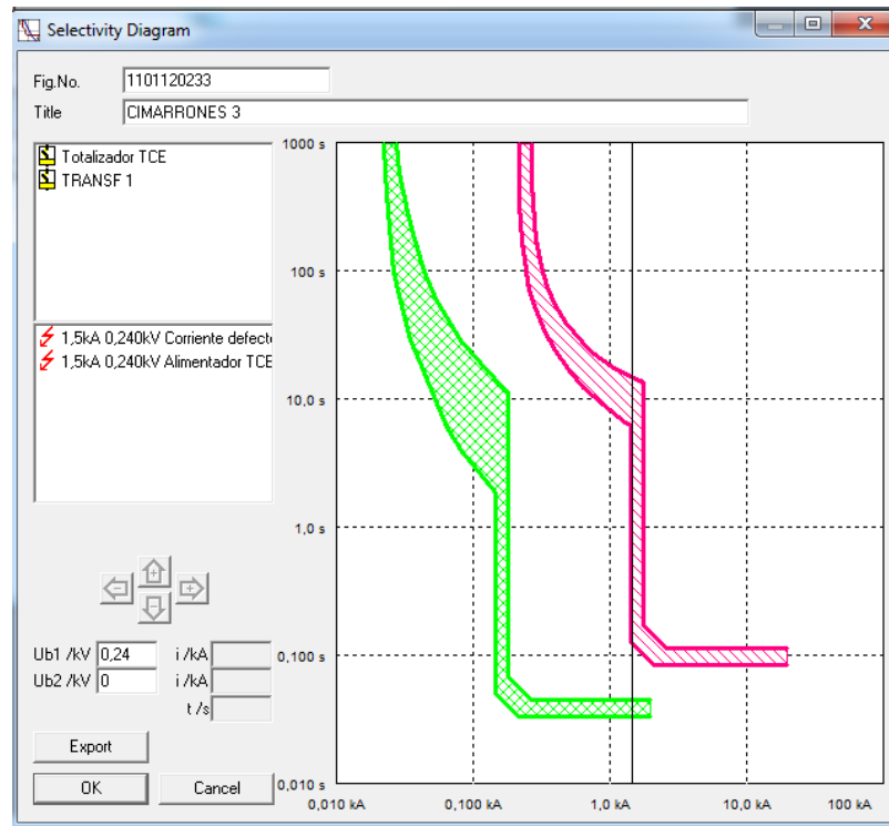
Grafica 4 Coordinación de la protección de cargas esenciales y protección de red normal de transferencia
