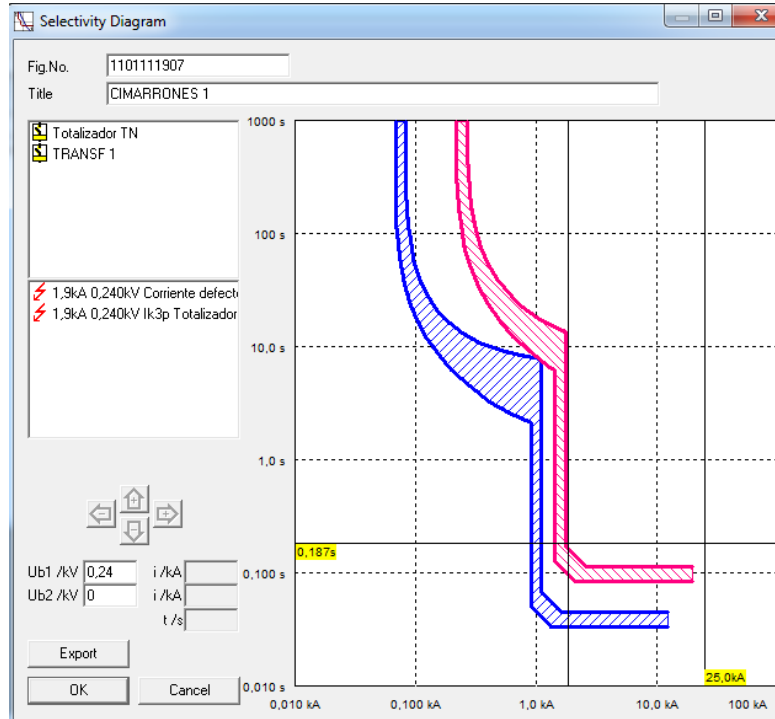
Grafica 2 Coordinación de la protección del tablero normal del primer piso y protección de red normal de transferencia
