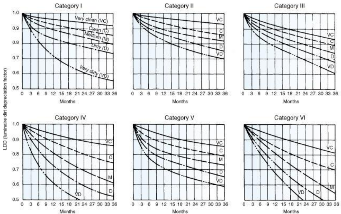
Grafica 7 Curva de categoría de mantenimiento de luminarias
