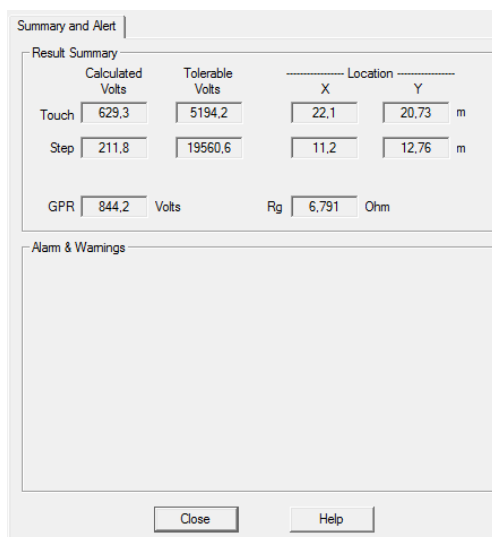
Figura 12 Resultados de resistencia de puesta a tierra y tensiones de paso y de contacto
