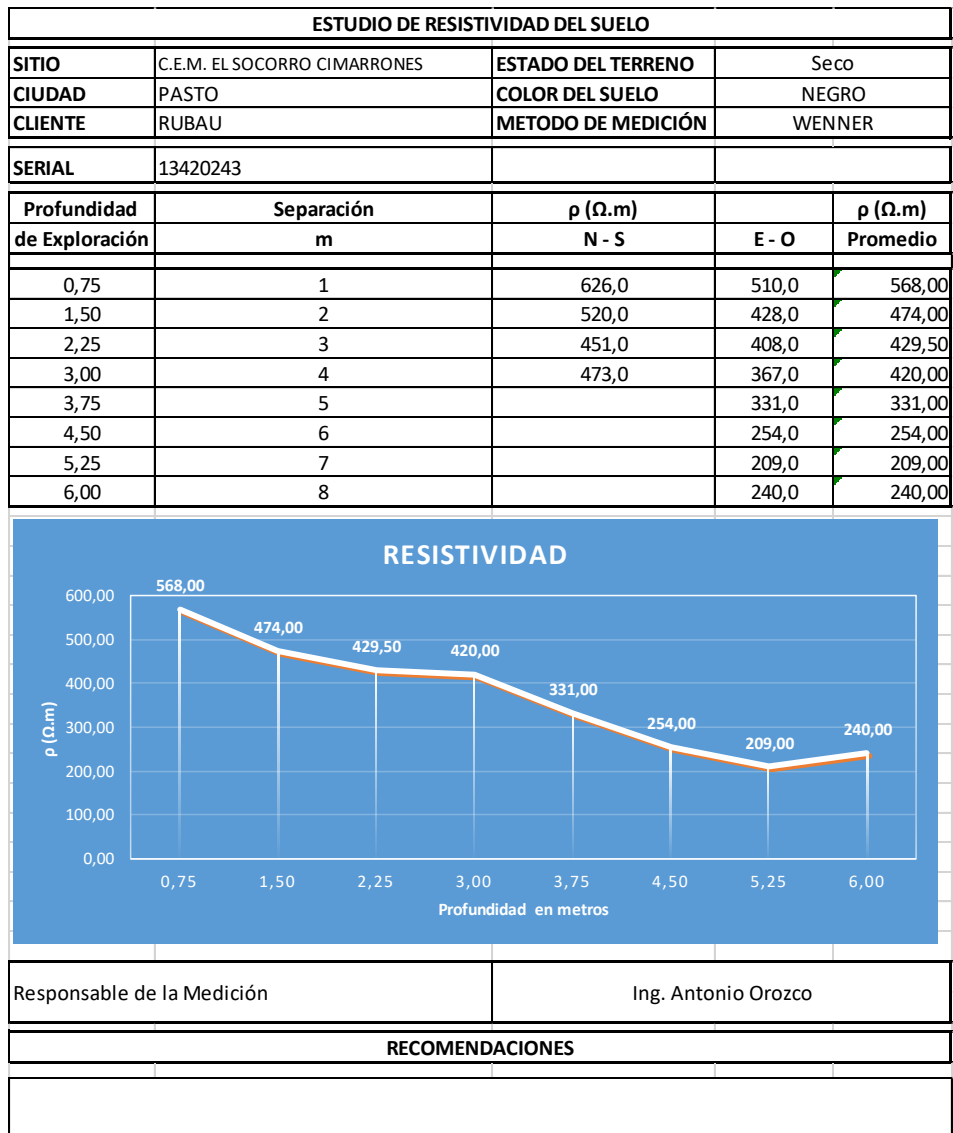
Grafica 6 Resultados de análisis de resistividad del terreno
