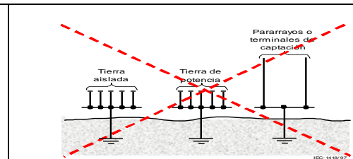
Figura 15.2. Puestas a tierra separadas o independientes
