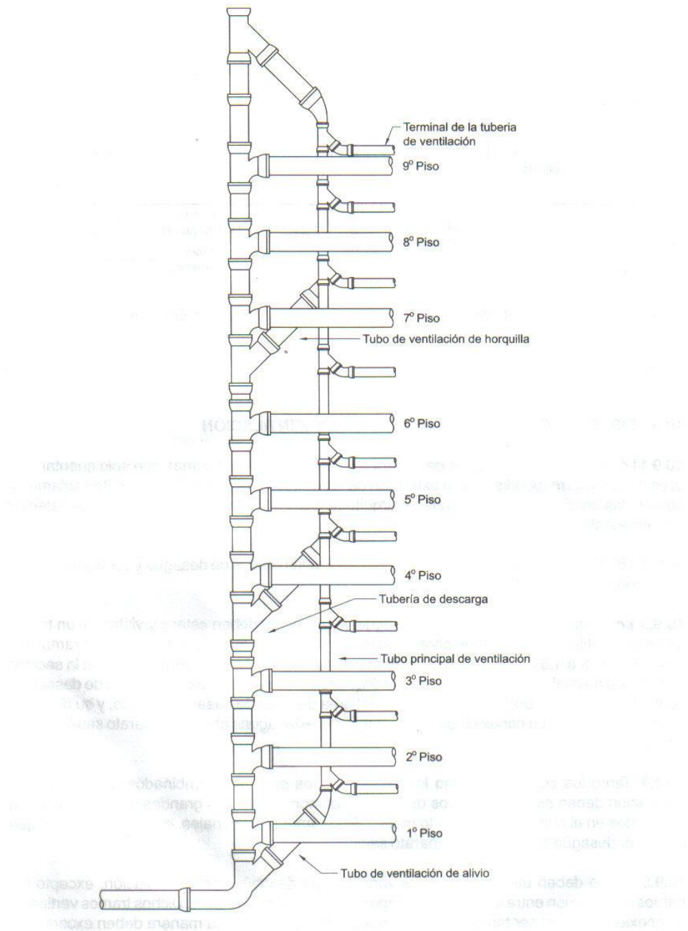
Figura 7. Conexión de ventilación de alivio ó de horquilla
