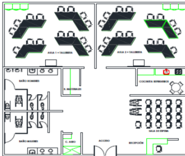
Fig. 1. Propuesta Arquitectónica de las intervenciones de Adecuaciones y/o Ampliaciones
