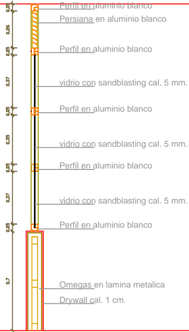
Detalle paneles Drywall-Vidrio-Persiana
