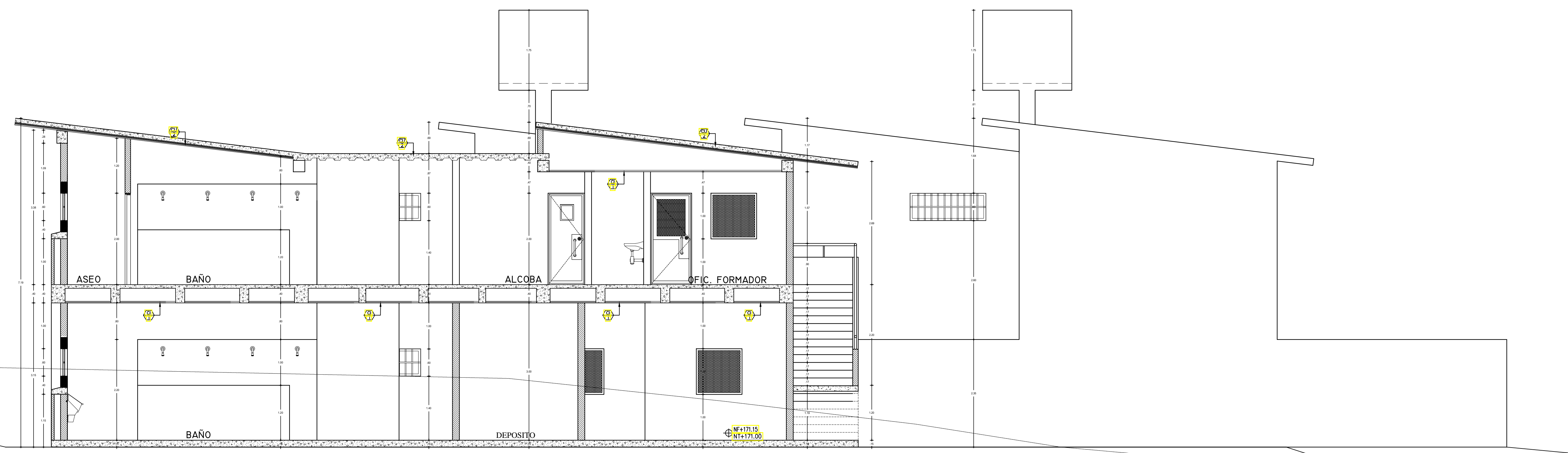
CORTE C - C'
