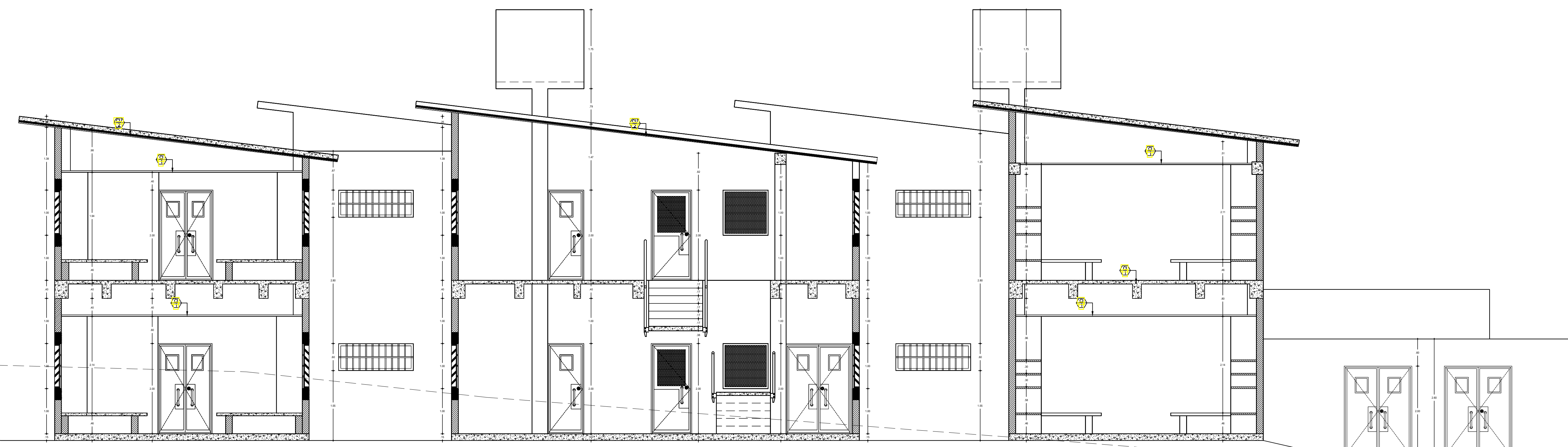
CORTE B - B'
