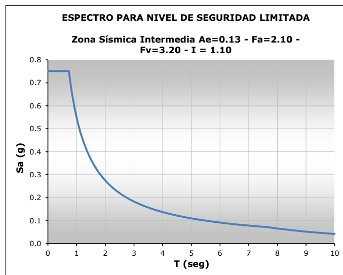
Figura 5. Espectro de Aceleraciones para un Nivel de Seguridad Limitada
