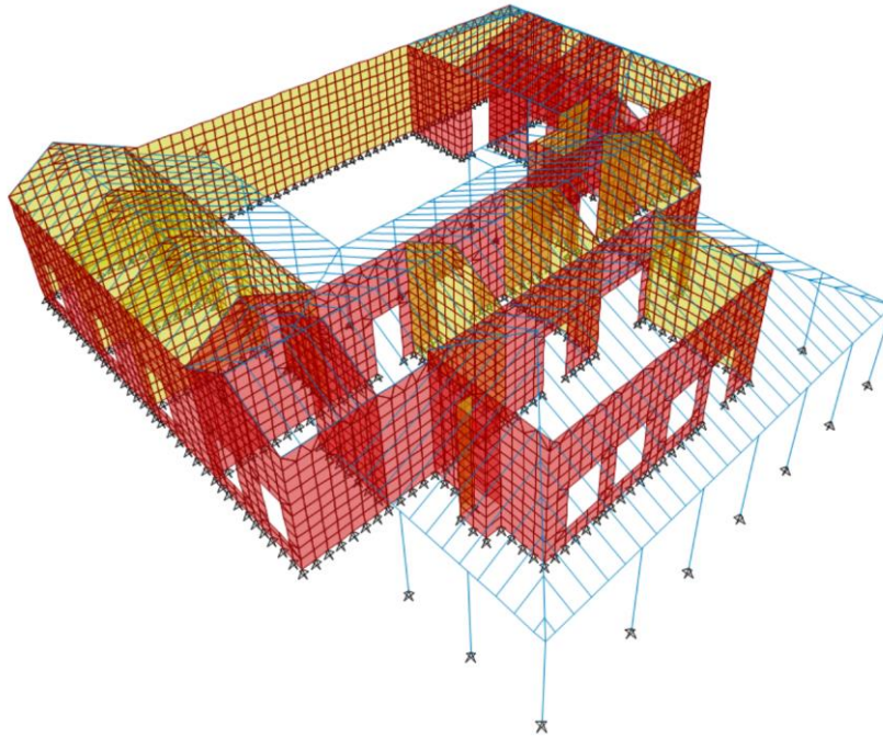
Figura 10. Modelo Computacional Tridimensional
