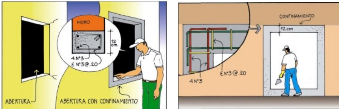
Figura 23. Esquema Reforzamiento Aberturas
