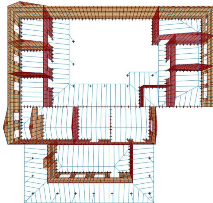
Figura 14. Modelo de análisis tridimensional - Planta
