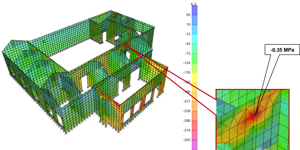
Figura 17. Esfuerzos Principales Mínimos (Compresiones) debido a Combinaciones Gravitacionales
