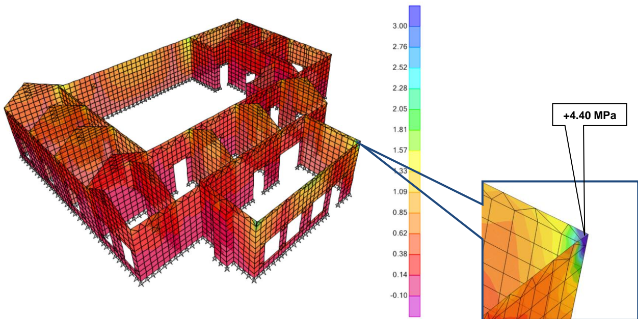
Figura 18. Esfuerzos Principales Máximos (Tracciones) debido a Combinaciones
