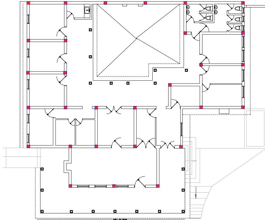
Figura 20. Localización propuesta de nuevas Columnas de Concreto
