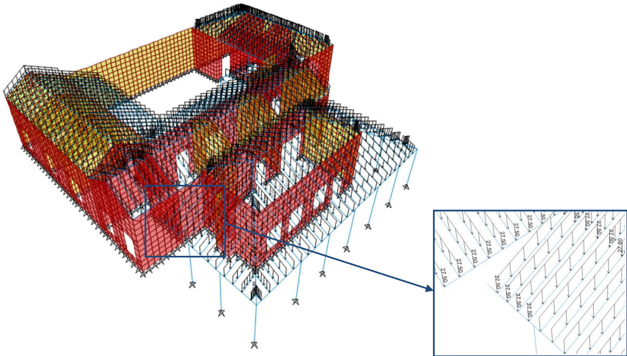
Figura 9. Cargas Vivas aplicadas al Modelo Computacional
