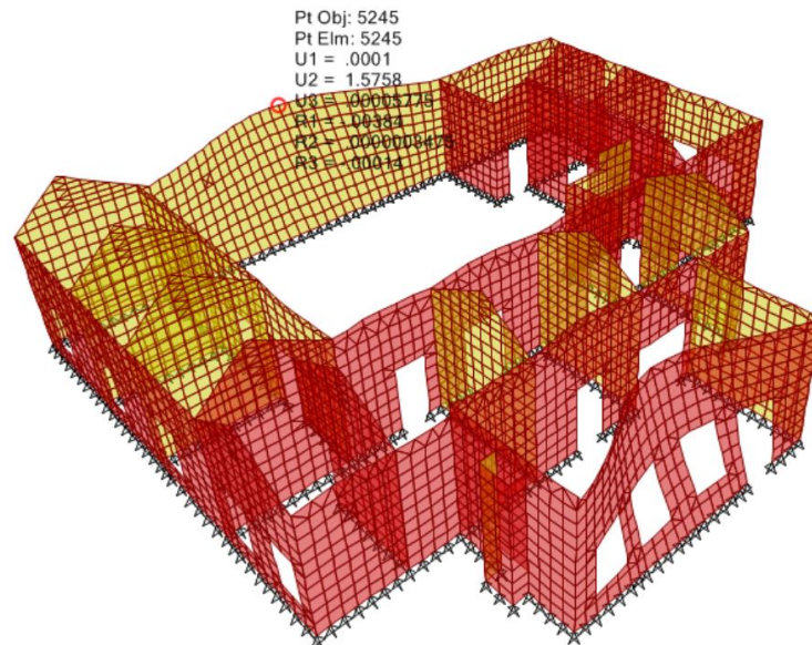
Figura 16. Desplazamientos originados por el Sismo en Dirección Transversal Y – Espectro Microzonificación
