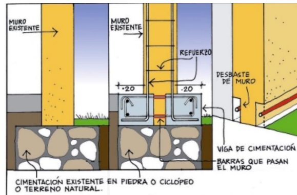
Figura 24. Esquema Refuerzo con Vigas de Cimentación
