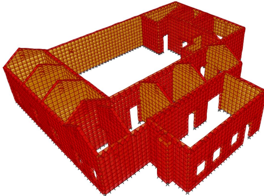
Figura 11. Modelo de Análisis Tridimensional Sistema Murario
