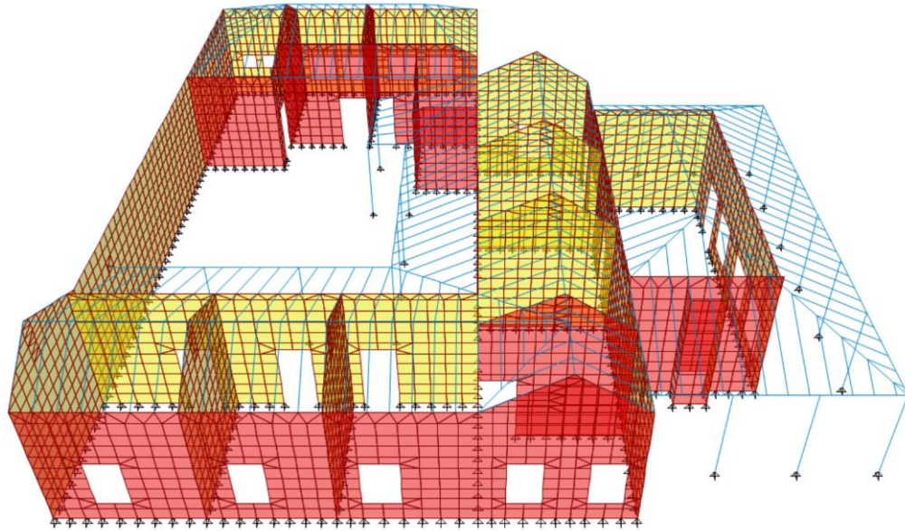
Figura 12. Modelo de análisis tridimensional - Vista Lateral
