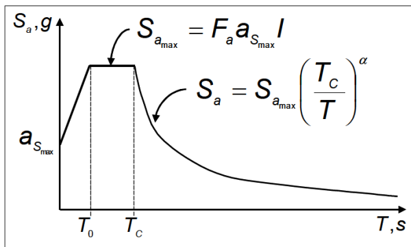
Figura 6. Espectro de Aceleraciones según Microzonificación Sísmica de Medellín
