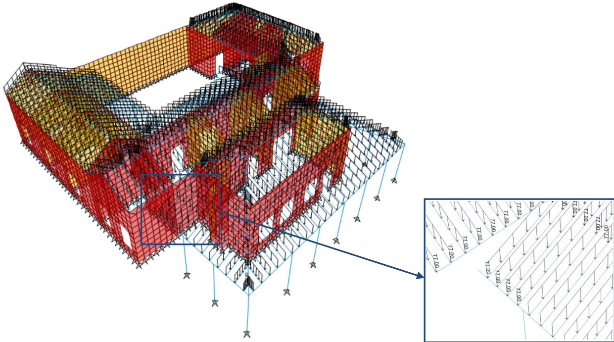
Figura 8. Cargas Muertas aplicadas al Modelo Computacional
