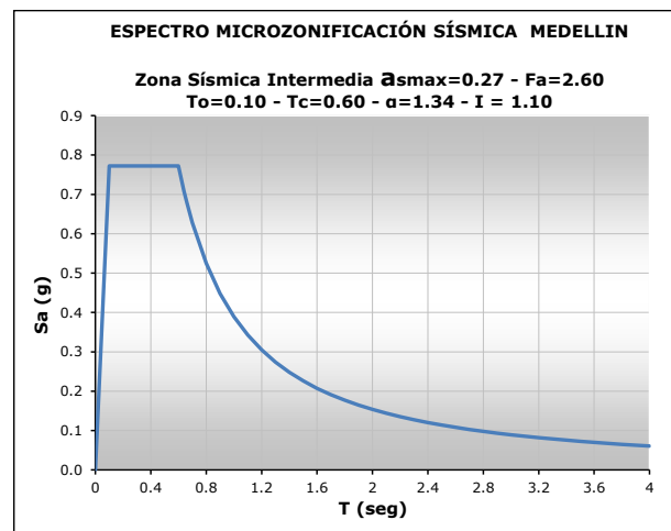
Figura 6. Espectro de Aceleraciones según Microzonificación Sísmica de Medellín
