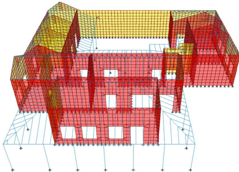
Figura 13. Modelo de análisis tridimensional - Vista Frontal
