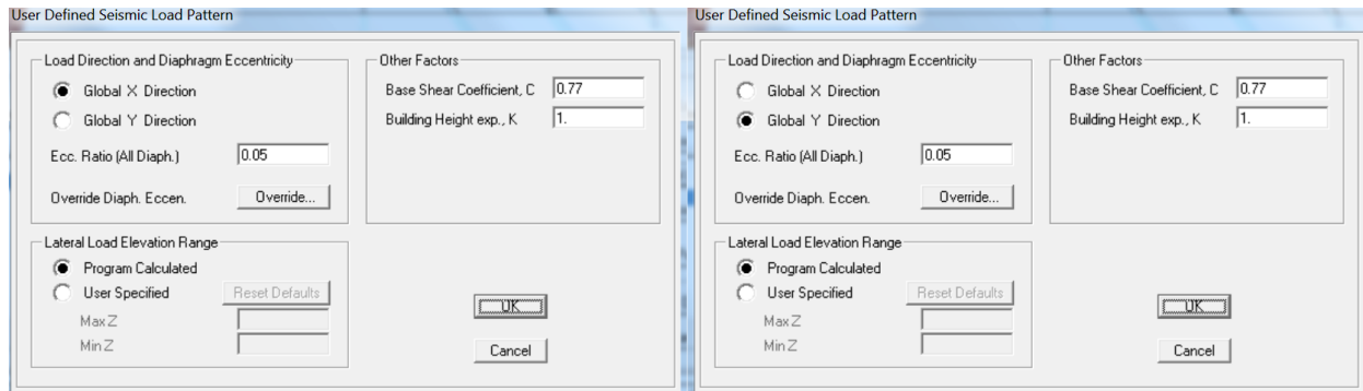
Figura 7. Asignación de los coeficientes por el MFHE – Espectro Microzonificación Medellín
