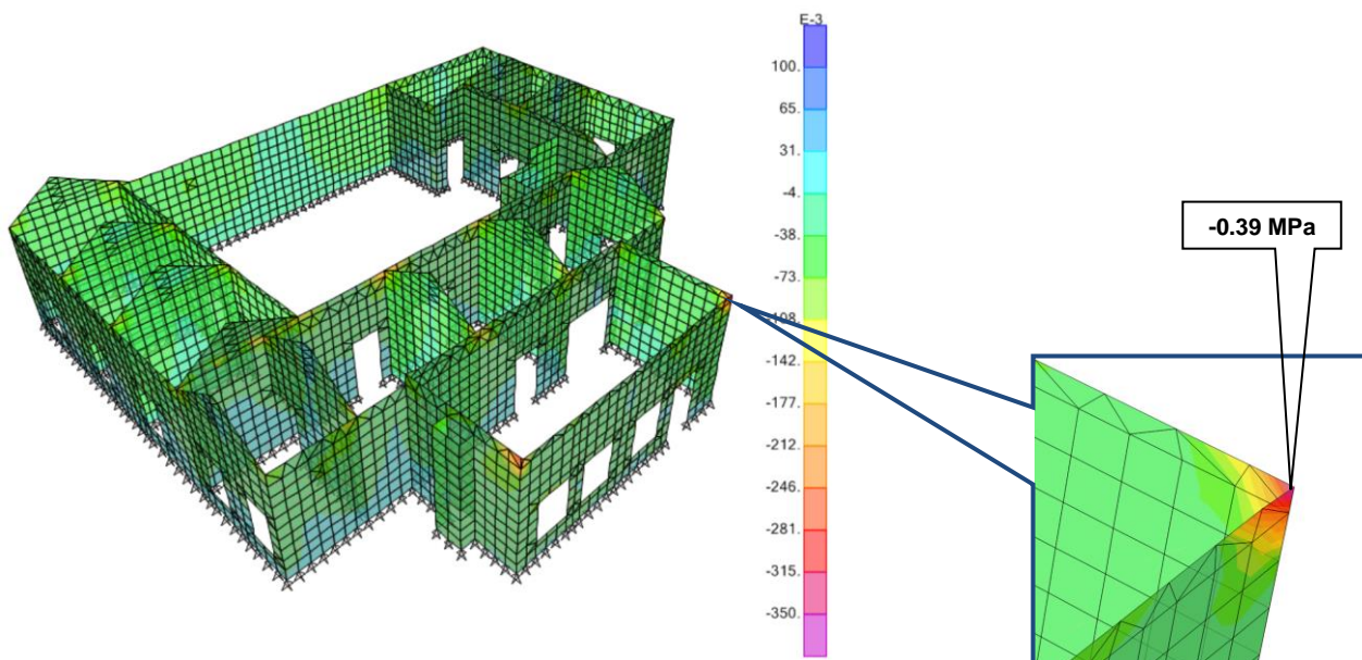
Figura 19. Esfuerzos Cortantes Máximos debido a Combinaciones Sísmicas
