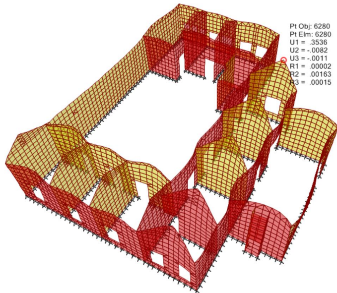
Figura 15. Desplazamientos originados por el Sismo en Dirección Longitudinal X – Espectro Microzonificación
