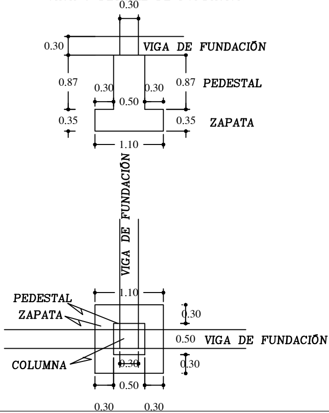
CASA 5 DETALLE DE FUNDACIÓN
