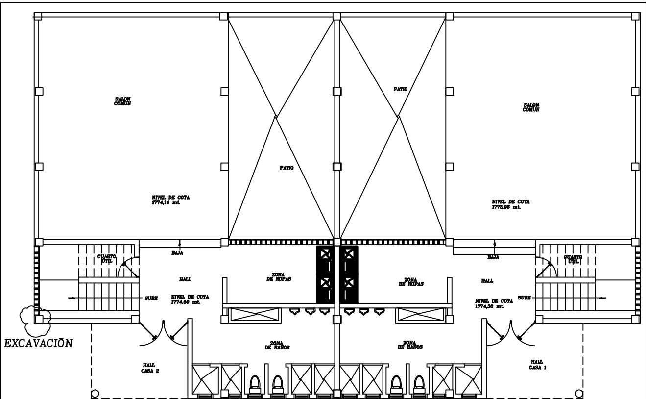
PLANTA PRIMER PISO CASA 5 SEDE SANTA RITA
