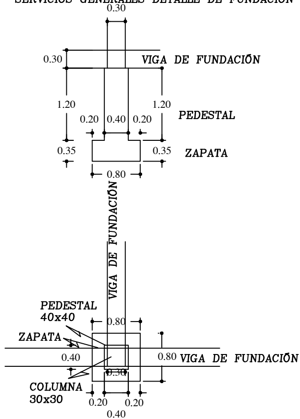
SERVICIOS GENERALES DETALLE DE FUNDACIÓN
